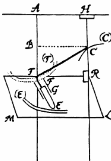
Principe d'un intégraphe universel, proposé par Leibniz (1693, trad. fcs. 1989 ; cité par Tournès). L'article de Coriolis se rattache clairement à cette méthode.
