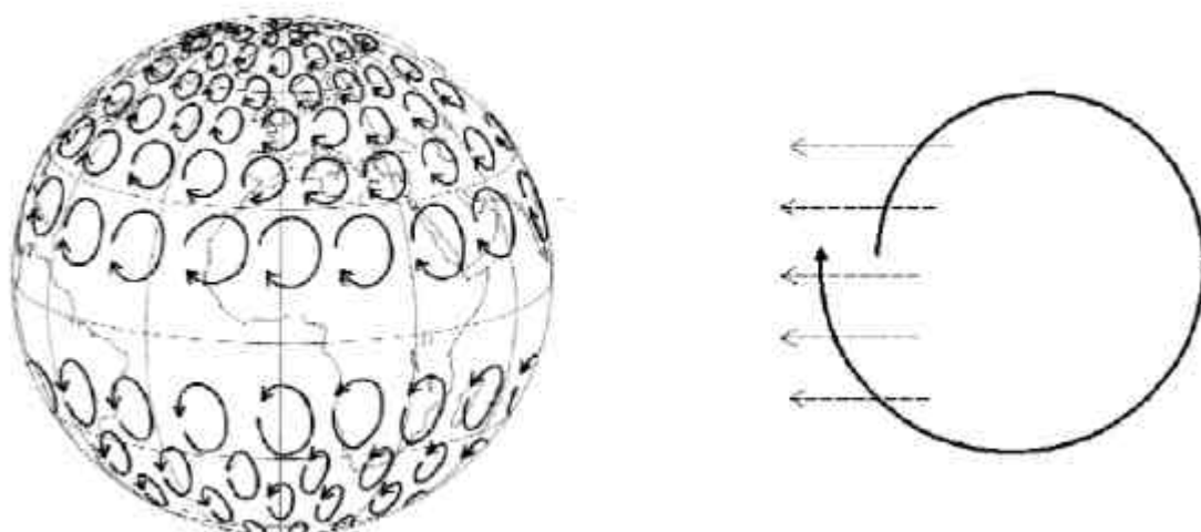
Extrait de l'article de Persson [2005], représentation en météorologie du mouvement circulaire inertielle dû à la force de Coriolis.
