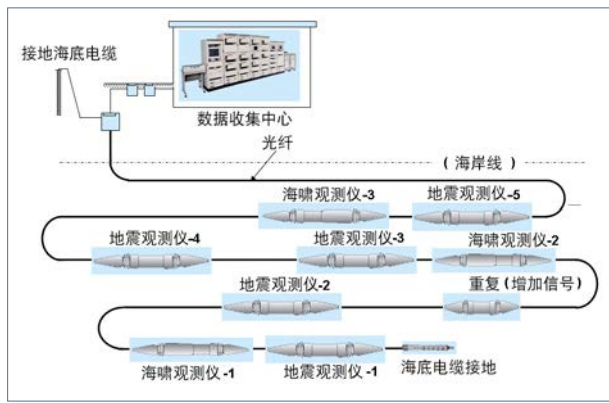
监测地震和海啸的海底电缆系统原理图。日本气象厅供图。
