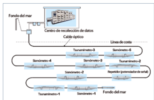
Diagrama esquemático del sistema de cableado oceánico desarrollado para el monitoreo de terremotos y tsunamis. Cortesía del JMA.
