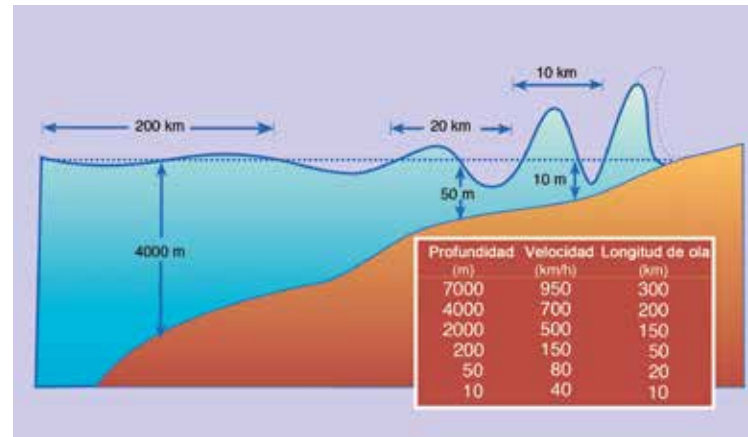
Altura de la onda y profundidad del agua. En aguas profundas, a menudo un tsunami tiene solo decenas de centímetros de altura, pero ésta crece rápidamente en aguas someras. La energía de la onda de un tsunami se extiende desde la superficie hasta el fondo en aguas profundas. Cuando un tsunami impacta contra la costa, la energía de la onda se concentra en una distancia menor creando ondas destructivas.
