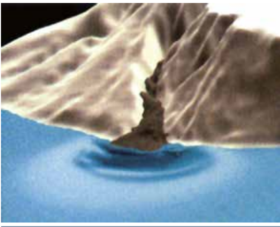
Los tsunamis pueden ser generados por flujos piroclásticos asociados a erupciones volcánicas. Cortesía de LDG (Francia).
