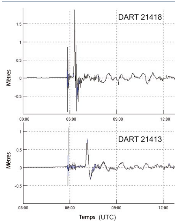
Enregistrement du tsunami du 11 mars 2011 par la bouée DART® #21418 située à 450 milles nautiques au nord-ouest de Tokyo. L'amplitude maximale de l'onde a été mesurée à 1,8 m, 33 minutes après le séisme. Le premier enregistrement correspond à la secousse due au séisme. Données reproduites avec l'autorisation de la NOAA
