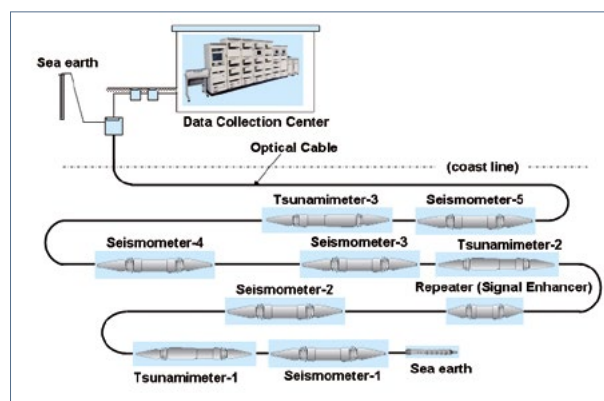
Schéma d'un système câblé océanique pour le suivi des séismes et des tsunamis. Avec l'autorisation du JMA Crédit image : Office météorologique japonais
