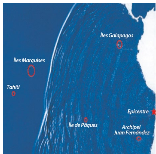
Modèle de propagation d'un tsunami dans le Pacifique Sud-Est, neuf heures après sa formation. Source : Antofagasta, Chili [30 juillet 1995]. Avec l'autorisation du LDG-France
