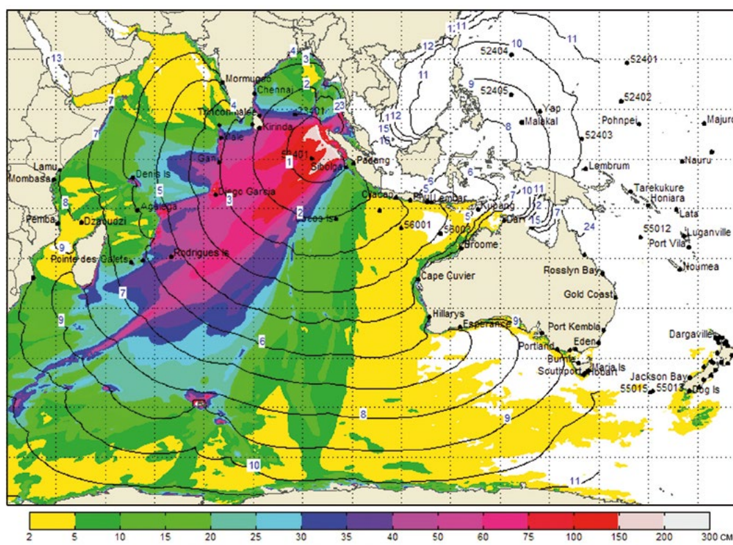
Carte de menace de tsunami établie par le RTSP australien de l'IOIWS pour l'océan Indien en fonction du séisme de magnitude 9,1 survenu le 26 décembre 2004 au large de Sumatra, Indonésie. Cette prévision aurait été émise si des centres internationaux d'alerte avaient été opérationnels en 2004. Les bandes colorées représentent les directions de propagation de l'énergie du tsunami et les amplitudes maximales au large des côtes. Les lignes de contour prévues indiquent le temps de parcours du tsunami à intervalle d'une heure. Avec l'autorisation du Centre australien conjoint d'alerte aux tsunamis.
