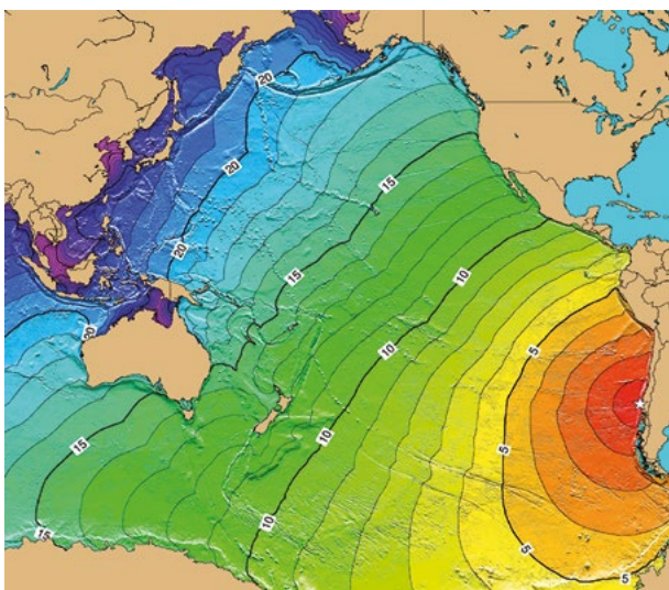
Temps de parcours (en heures) du tsunami du 22 mai 1960 qui, depuis le Chili, a traversé tout le Pacifique. Il a provoqué d'énormes dégâts le long de la côte voisine du Chili, causé de nombreuses destructions et fait des victimes jusqu'à Hawaii et au Japon. La prise de conscience et l'inquiétude que ce tsunami à l'échelle du Pacifique a suscitées ont finalement conduit à la création du PTWS. Crédit image : CIIT.
