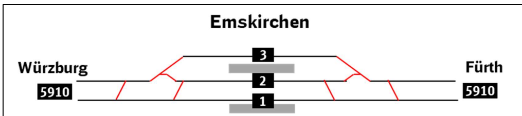
Abbildung 41: Mittiges Überholungsgleis in Emskirchen
