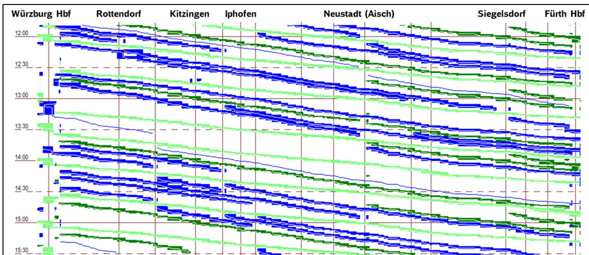
Abbildung 49: Ausgeprägter Mischverkehr auf der Strecke Fürth - Würzburg
