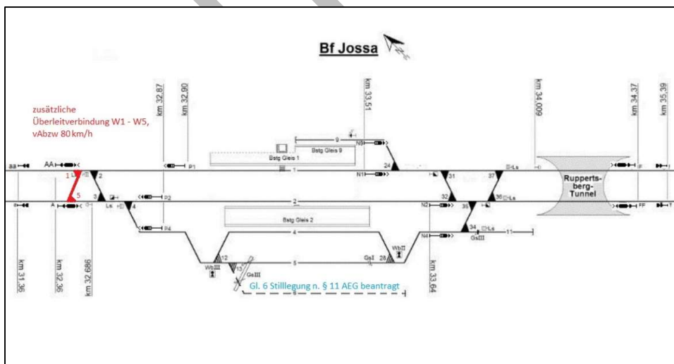
Abbildung 30: Zusätzliche Weichenverbindung im Bahnhof Jossa
