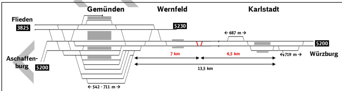
Abbildung 34: Spurplanskizze Bahnhof Karlstadt
