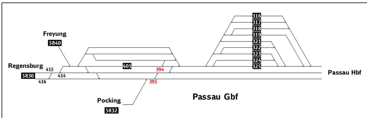
Abbildung 46: Erhöhung der Überleitgeschwindigkeit an Weichen im Bereich von Passau Gbf
