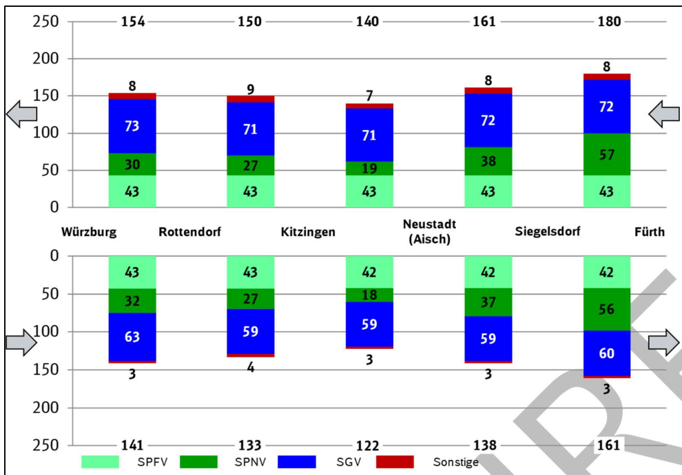
Abbildung 10: Abschnittsbezogene Zugzahlen nach Verkehrsarten am 25.03.2021
