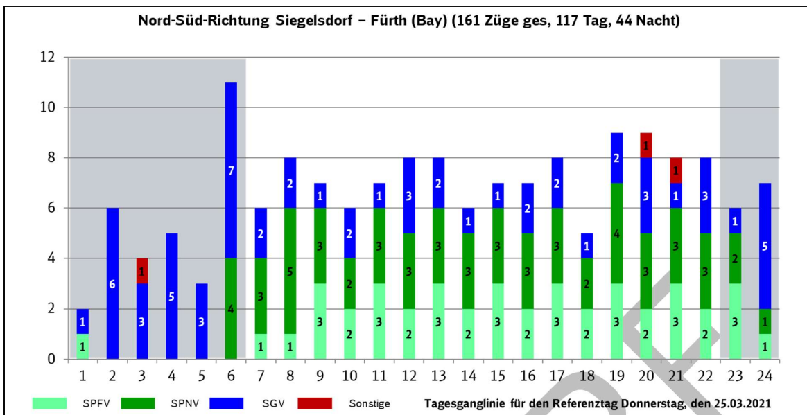
Abbildung 12: Tagesganglinie für Donnerstag, 25.03.2021 - von Siegelstorf nach Fürth (Bay)
