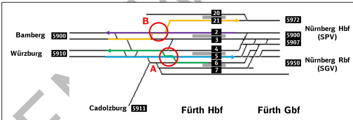
Abbildung 27: Weitere niveaugleiche Fahrwegkreuzungen in Fürth Hbf
