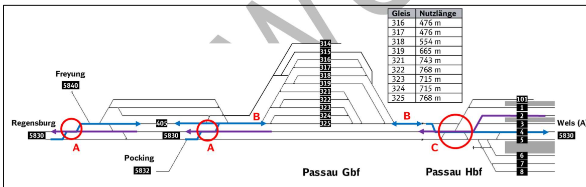
Abbildung 28: Kapazitätsbeschränkende Punkte im Bereich Passau Hbf/Gbf
