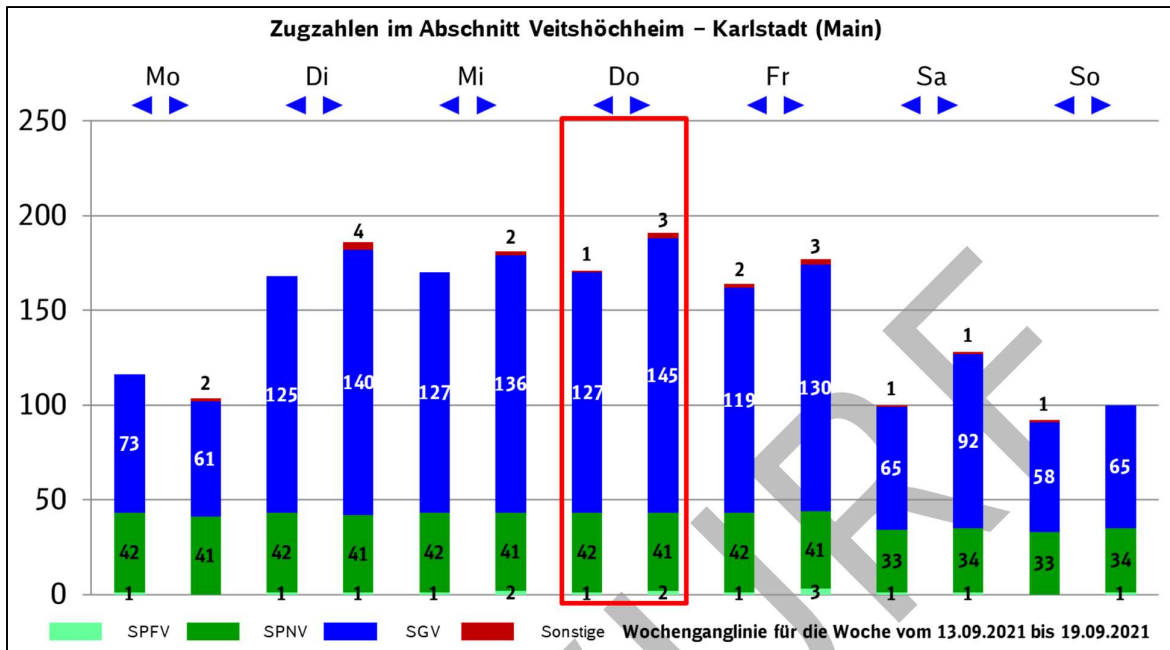
Abbildung 7: Wochenganglinie des Abschnitts Veitshöchheim – Karlstadt (Main)
