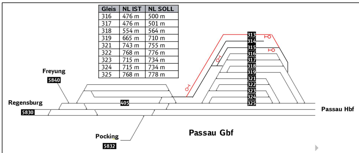
Abbildung 48: Erhöhung der Abstellkapazität in Passau Gbf
