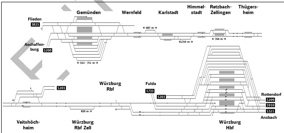
Abbildung 3: Streckenübersicht Gemünden – Würzburg Hbf
