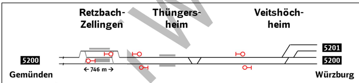
Abbildung 36: Anpassungen im ESTW-Bereich Retzbach-Zellingen - Thüngersheim
