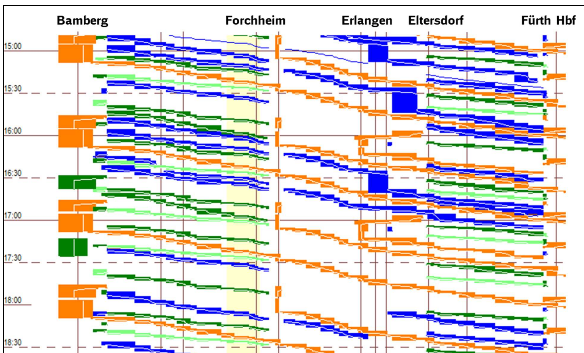
Abbildung 20: Fahrplanstruktur zwischen Bamberg und Fürth
