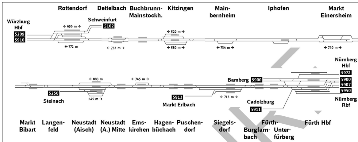
Abbildung 4: Streckenübersicht (Würzburg Hbf -) Rottendorf - Fürth Hbf
