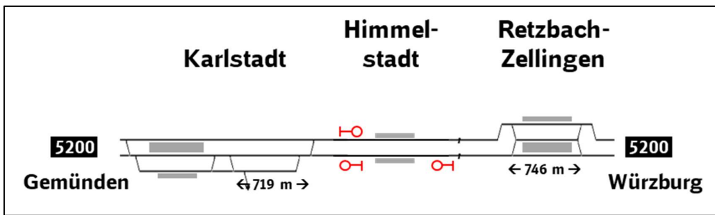
Abbildung 35: Zusätzliche Blocksignale im Abschnitt Retzbach-Zellingen - Karlstadt
