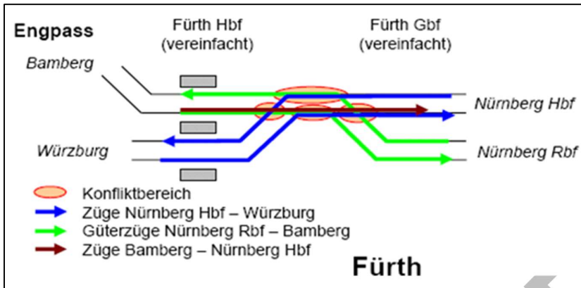
Abbildung 26: Niveaugleiche Kreuzung des SGV in der Relation Nürnberg Rbf - Bamberg
