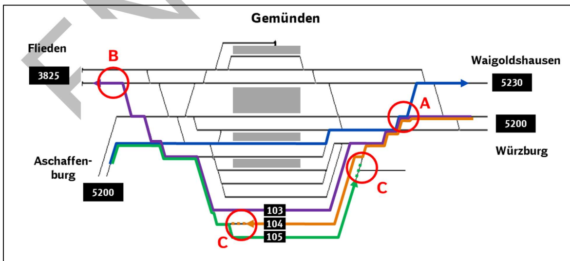
Abbildung 21: Kapazitätsmindernde Punkte im Bahnhof Gemünden
