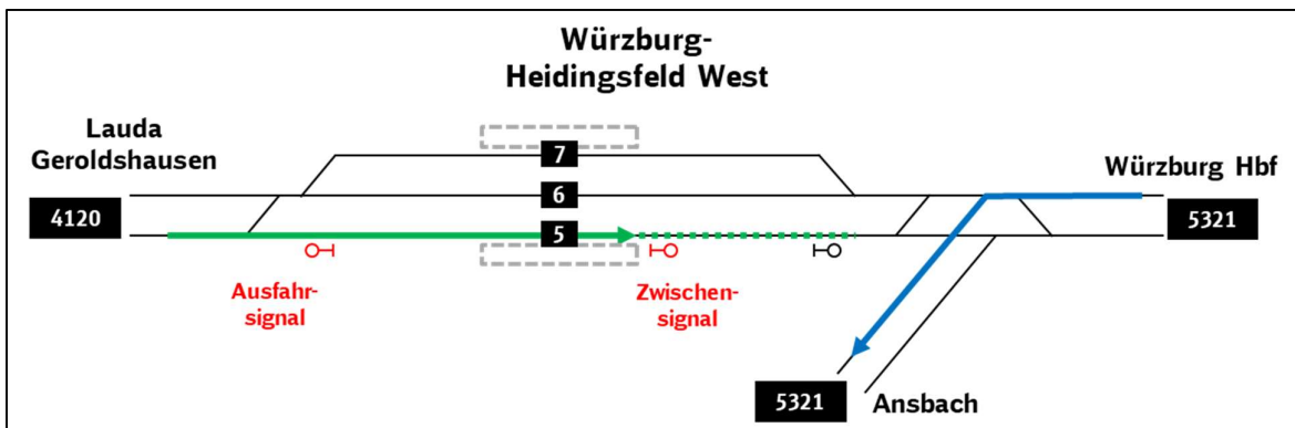
Abbildung 37: Zusätzliche Signale in Heidingsfeld West
