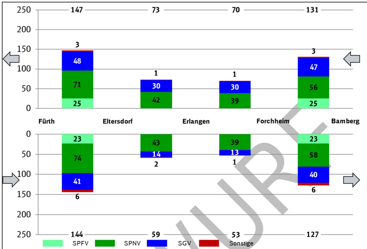
Abbildung 14: Abschnittsbezogene Zugzahlen nach Verkehrsarten am 02.06.2021
