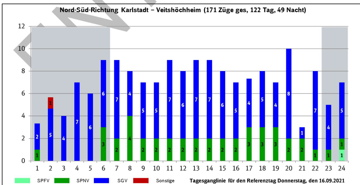
Abbildung 8: Tagesganglinie für Donnerstag, 16.09.2021 - von Karlstadt nach Veitshöchheim
