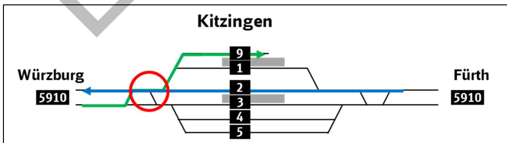
Abbildung 24: Fahrstraßenausschlüsse in Kitzingen
