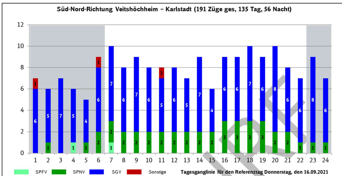
Abbildung 9: Tagesganglinie für Donnerstag, 16.09.2021 - von Veitshöchheim nach Karlstadt
