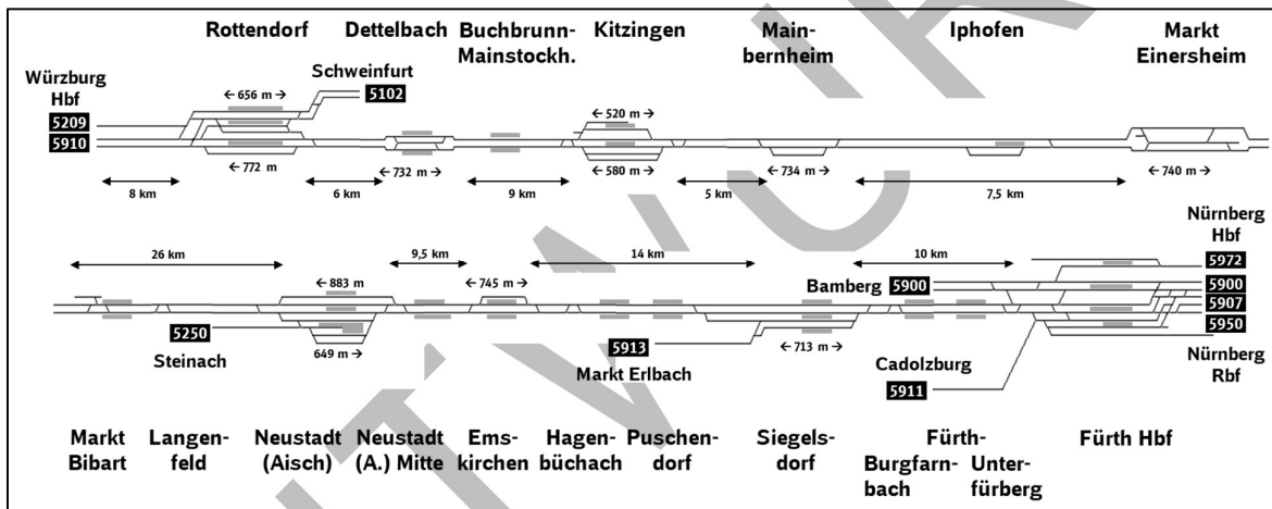
Abbildung 23: Streckenübersicht mit den Abständen der Überholungsmöglichkeiten zwischen Würzburg Hbf und Fürth Hbf
