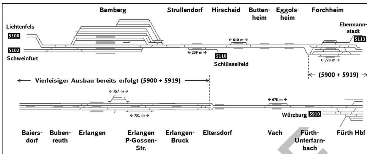
Abbildung 5: Streckenübersicht Bamberg - Fürth Hbf
