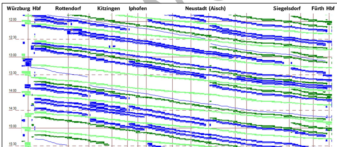
Abbildung 19: Fahrplanstruktur zwischen Würzburg und Fürth
