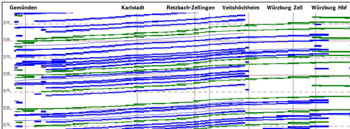
Abbildung 18: Fahrplanstruktur zwischen Gemünden und Würzburg
