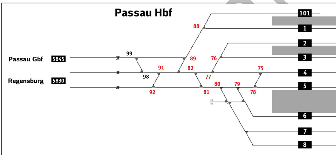
Abbildung 47: Erhöhung der Überleitgeschwindigkeit an Weichen im Westkopf von Passau Hbf
