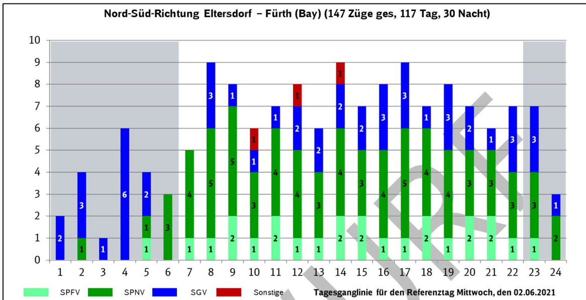
Abbildung 16: Tagesganglinie für Mittwoch, 02.06.2021 - von Eltersdorf nach Fürth (Bay)
