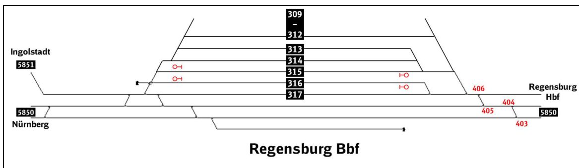
Abbildung 45: Erhöhung der Überleitgeschwindigkeit und zusätzliche Hauptsignale in Regensburg Bbf
