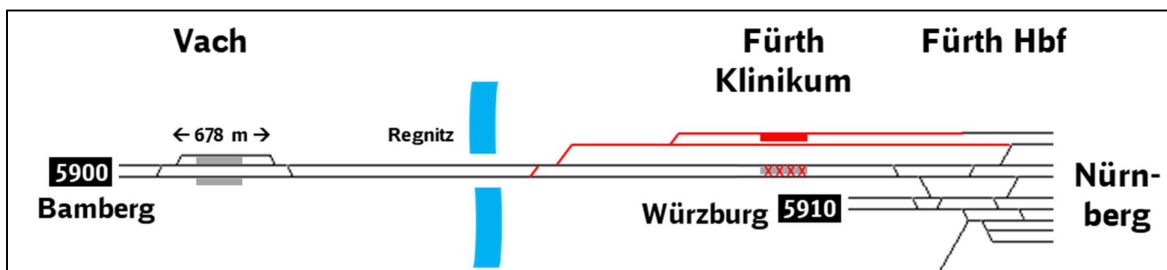
Abbildung 42: Zusätzliche S-Bahn-Gleise nördlich von Fürth Hbf
