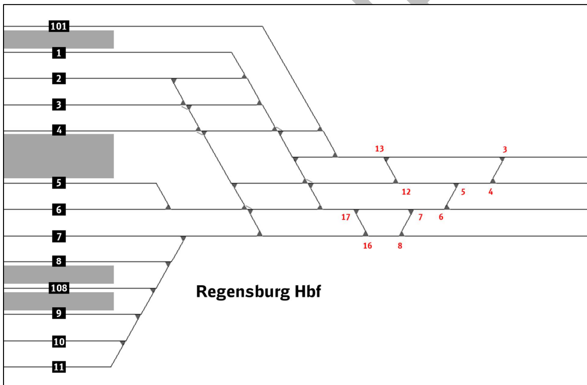
Abbildung 44: Erhöhung der Überleitgeschwindigkeit an Weichen im Ostkopf von Regensburg Hbf
