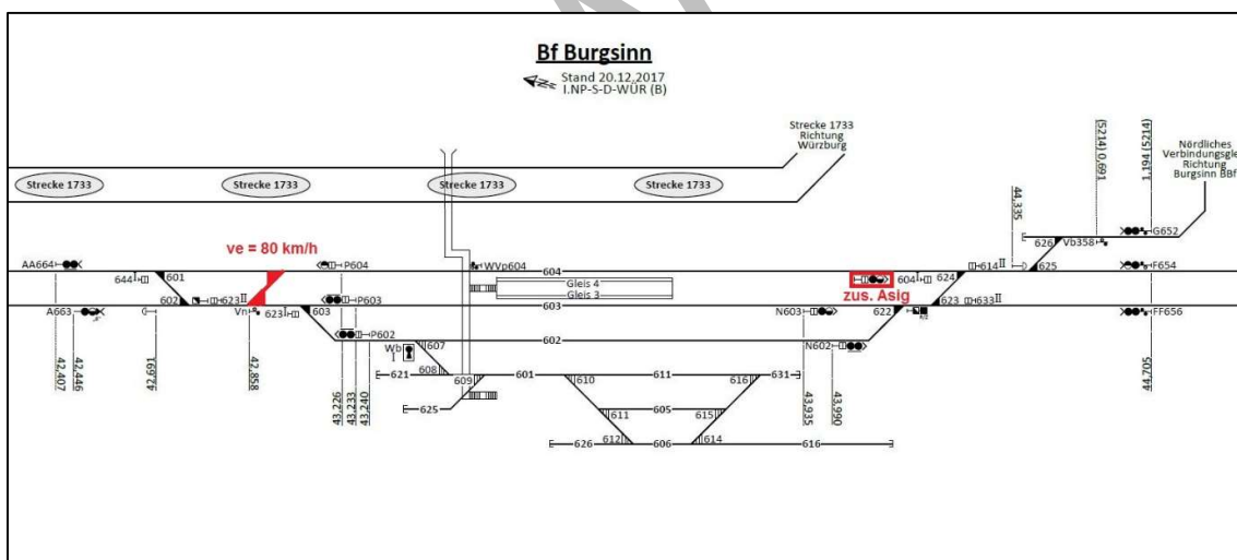
Abbildung 31: Zusätzliche Weichenverbindung und zusätzliches Ausfahrtsignal Burgsinn
