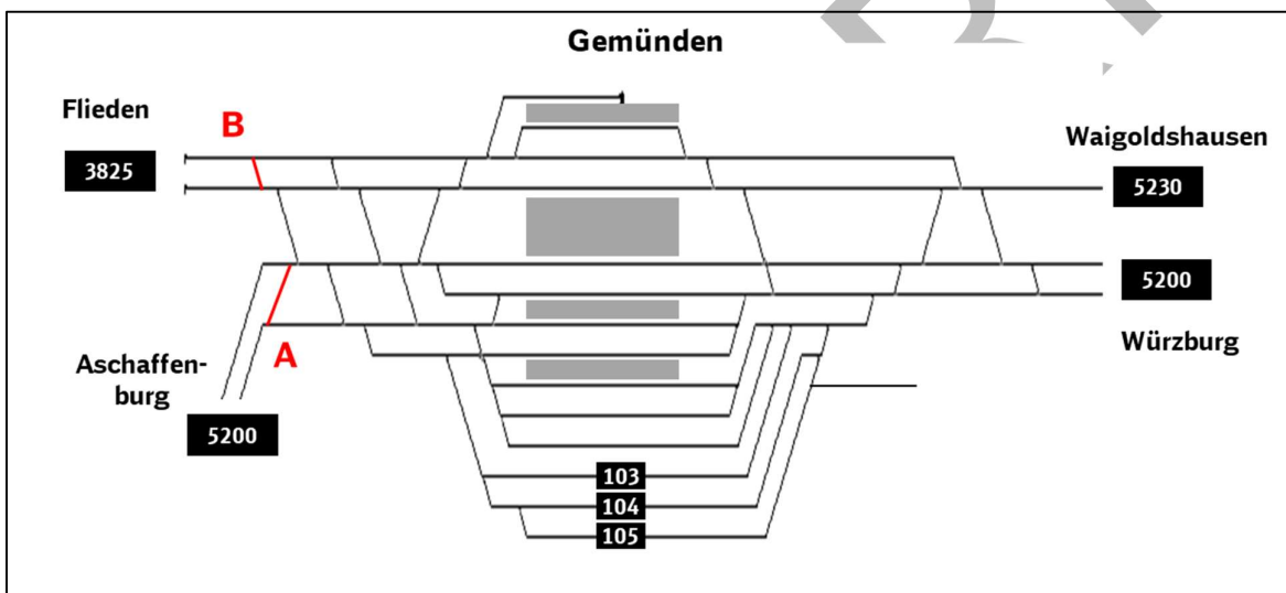
Abbildung 32: Zusätzliche Weichenverbindungen im nordwestlichen Bahnhofskopf Gemünden (Main)
