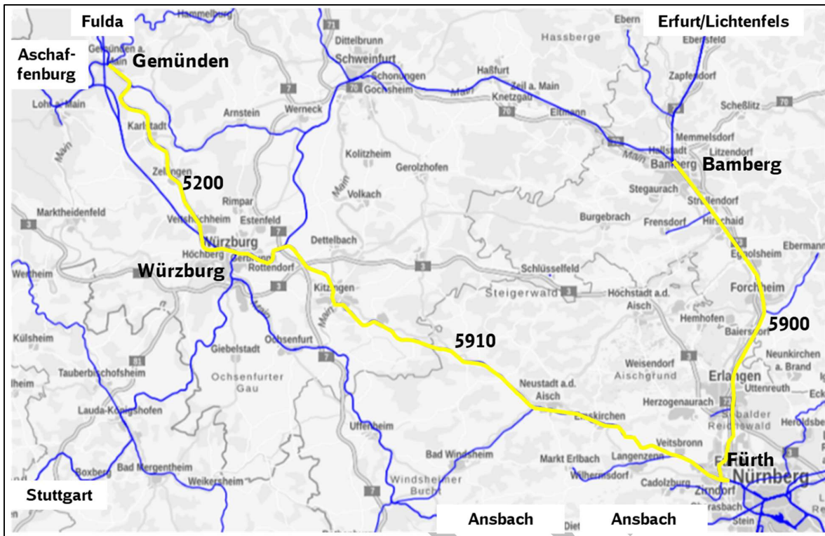
Abbildung 2: Die Lage im Netz der überlasteten Strecken
