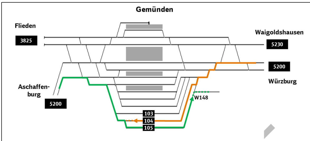
Abbildung 33: Zusätzlicher Durchrutschweg für die Einfahrt nach Gleis 105 im Bahnhof Gemünden (Main)
