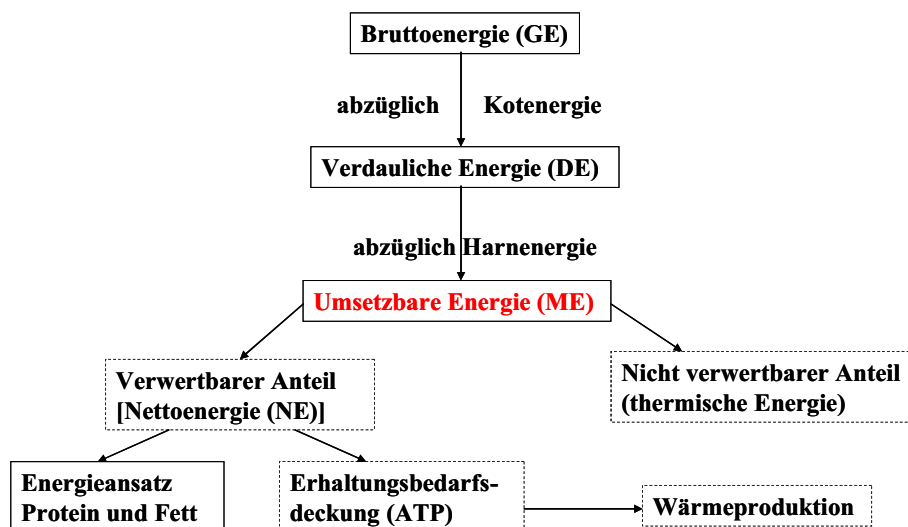
Abb. 5.1.1: Energienstufen
