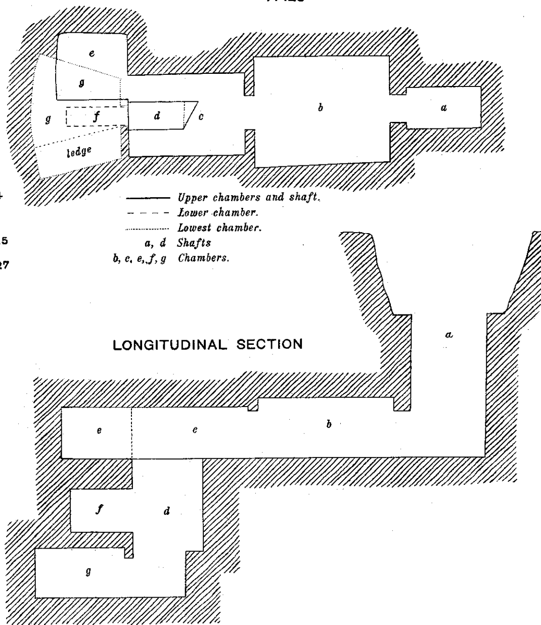
PLAN 1:125
