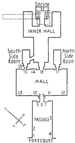
Asyût. Tomb 1. Hepzefa I. From Descr. de l'Égypte, Ant. iv, pl. 44 [1].
