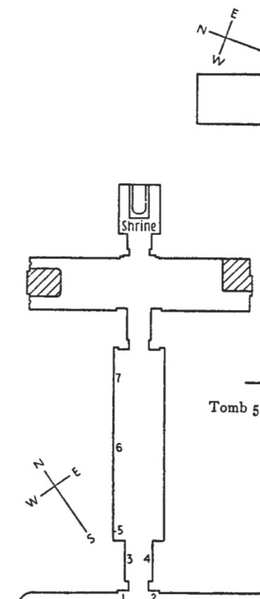
Tomb 3. Aḥmosi. From DAVIES, iii, pl. xxvi.
