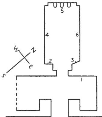
EL-SIRÎRÎYA. Rock-chapel. From L. D. Text , ii, p. 47.
