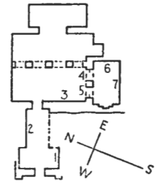
EL-KÔM EL-AḤMAR. Ni'ankh-Pepy. From L. D. i. 57 [Tomb 14].
