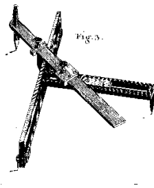
Fig. 55: Halbellipsenzirkel nach Adams
