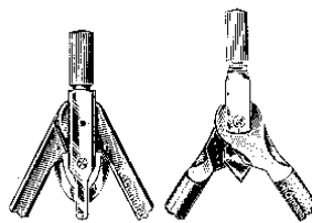
Fig. 14: Starrer und beweglicher Griff; Katalog Fa. Wichmann
