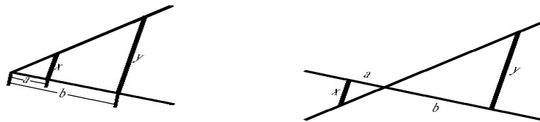
Fig. 35: Strahlensatzfiguren
