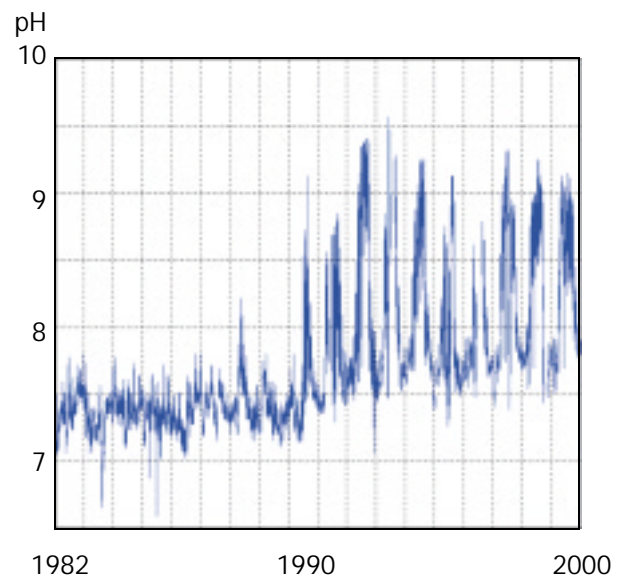
Abb. 5.2: pH-Wert-Ganglinie der Elbe bei Schnackenburg 1982 - 1999
