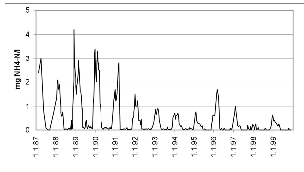
Abb. 5.6: Verlauf der Ammoniumgehalte an der Messstelle Grauerort (km 660,5)
