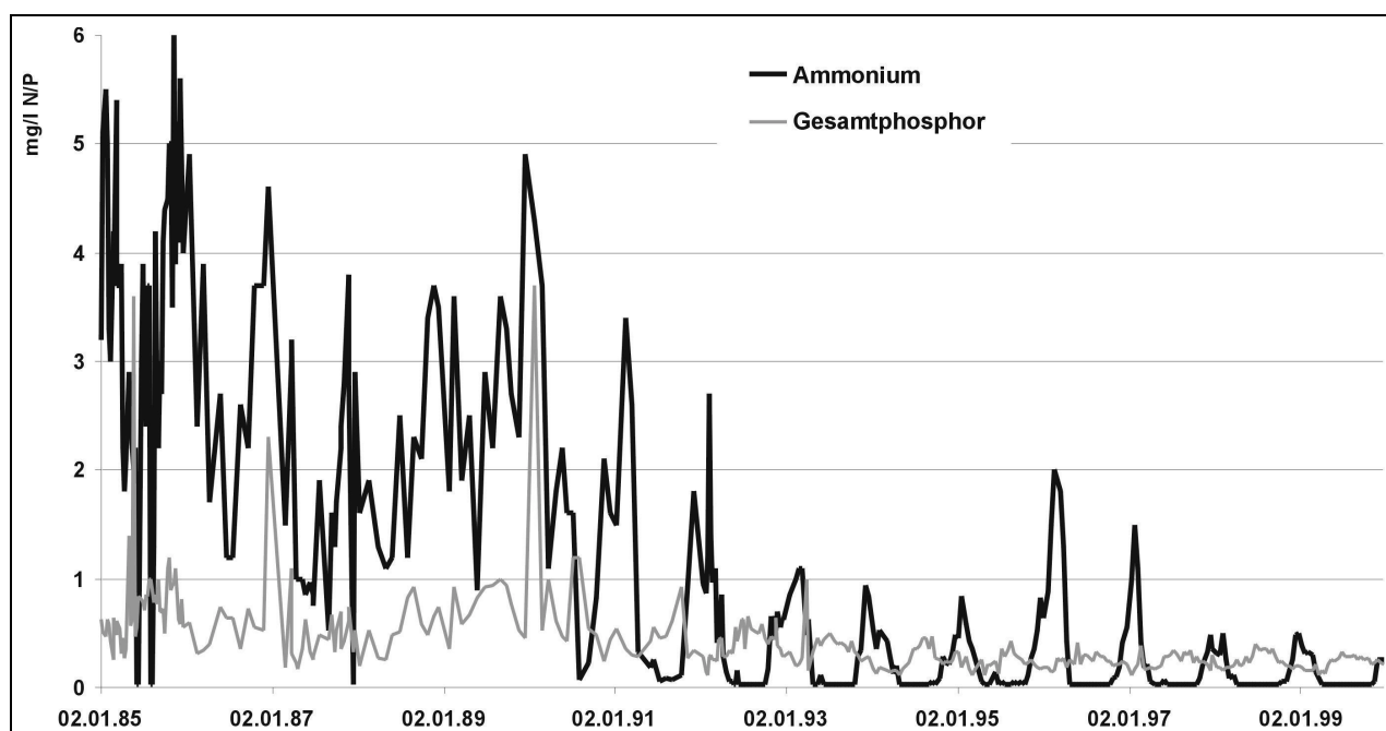
Abb. 5.3: Ammonium- und Gesamtphosphorkonzentrationen in der Elbe bei Schnackenburg von 1985 bis 1999
