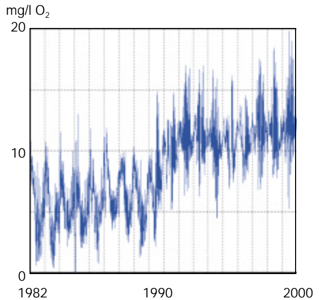
Abb. 5.1: Sauerstoffganglinie der Elbe bei Schnackenburg 1982 - 1999
