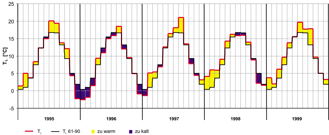
Abb. 3.1: Monatsmittel der Lufttemperatur T_L im Vergleich zum langjährigen Mittel in °C (aus Tagesmittelwerten des DWD an der Station Steinkirchen)
