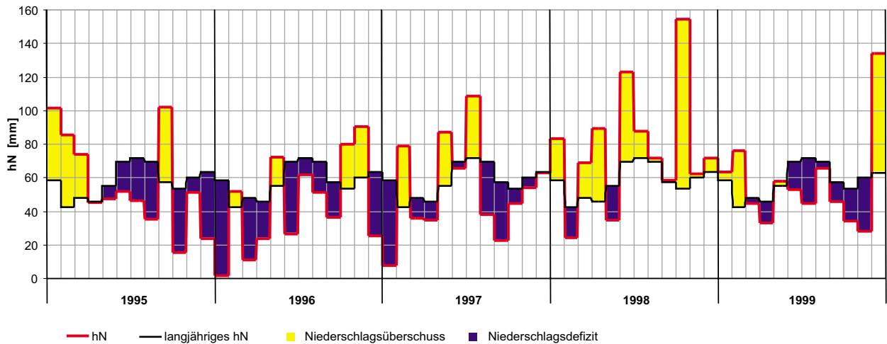
Abb. 3.2 Mittlere monatliche Niederschlagshöhen h_N im Berichtsgebiet im Vergleich zum langjährigen Mittel (Mittel der Gebietsniederschläge für Lüchow, Bienenbüttel, Jehrden und Rockstedt gem. DWD)
