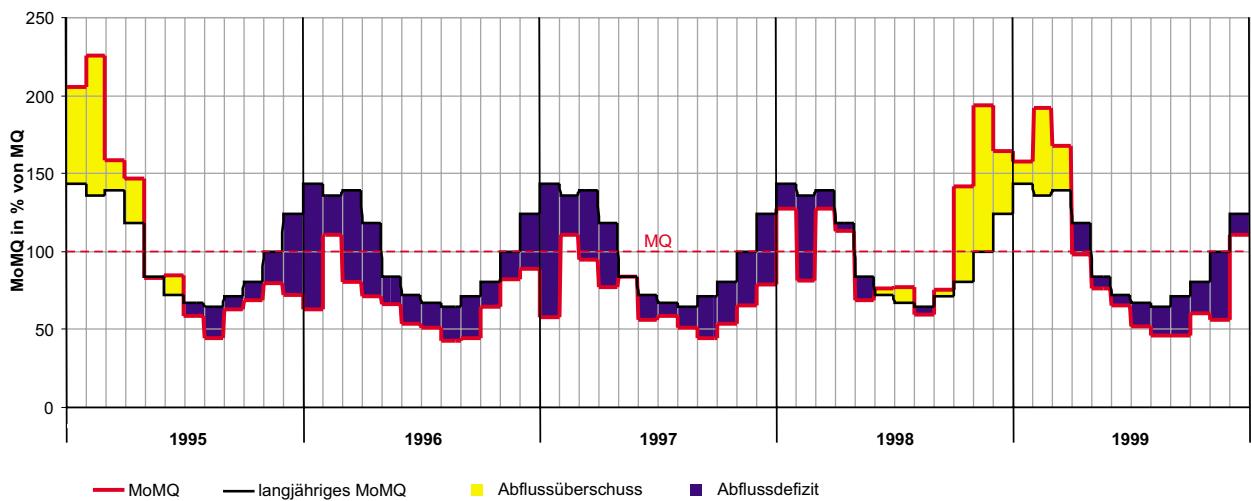
Abb. 3.3: Mittlere Abflüsse in % von MQ der Gewässer im Berichtsgebiet im Vergleich zum langjährigen Mittel (Mittel der Werte an den Pegeln Lüchow, Bienenbüttel, Jehrden und Rockstedt)
