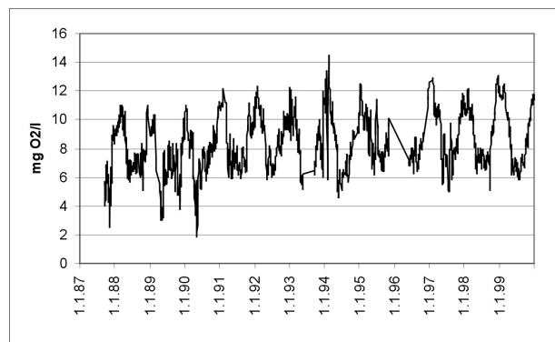
Abb. 5.7: Verlauf der Sauerstoffgehalte an der Messstation Grauerort (Tagesmittelwerte)
