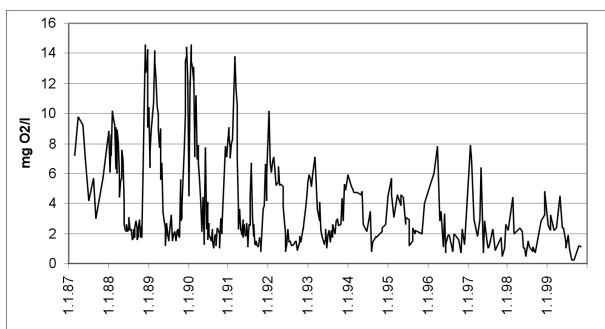
Abb. 5.5: Verlauf des Biochemischen Sauerstoffbedarfes (BSB 5 ) an der Messstelle Grauerort (km 660,5)
