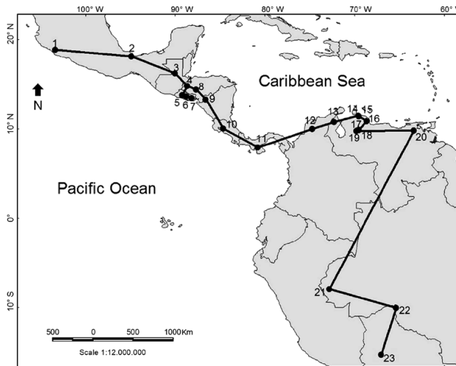
Figure 1. Geographic distribution of Mixotoxodon larensis in Central and South America. México: 1) Hihuitlán, Michoacan State; 2) La Estribera, Veracruz State. Guatemala: 3) Santa Amelia River, Petén department. Honduras: 4) Yeroconte, Lempira department. 8) Orillas del Humuya, Comayagua department. El Salvador: 5) Tomayate, San Salvador department; 6) Barranca del Sisimico, San Vicente department; 7) Hormiguero, San Miguel department. Nicaragua: 9) El Bosque, Estalí department. Costa Rica: 10) Bajo de los Barrantes, Alajuela province. Panamá: 11) Ocu, Herrera province. Colombia: 12) Chivolo, Magdalena department. Venezuela: 13) Mene de Inciarte in Zulia State; 14) Muaco, 15) Ocando, and 16) Cerro Misión, in Falcón State; 17) Agua Viva del Totumo; 18) San Miguel; and 19) El Tocuyo in Lara State; 20) El Breal de Orocuál, Monagas State. Brazil: 21) Juruá River, Acre State; 22) Araras/Periquitos Rondonia State. Bolivia: 23) Cara Cara, Beni department.
