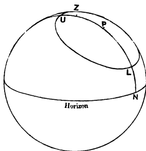
Fig. 6. Circumpolar Star.
