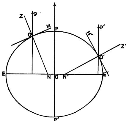
Fig. 8. Latitude on a Spheroidal Earth.
