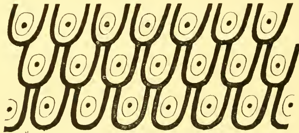
FIG. 150. SCALE-PATTERN (DAPHNAE).
