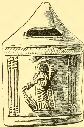
FIG. 200. TERRACOTTA MONEY-BOX.
