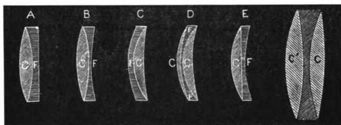
FIG. 324. ACHROMATIC LENSES.
