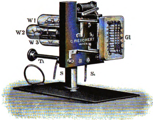
FIG. 54. NERNST LAMP FOR THE MAGIC LANTERN (REICHERT).
