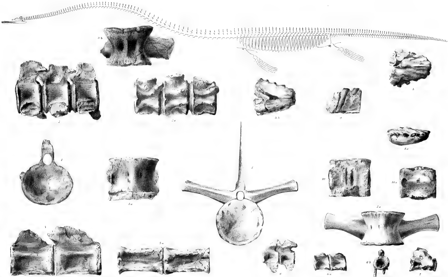
Figs 1-9 Ichthyosaurus platyrus
