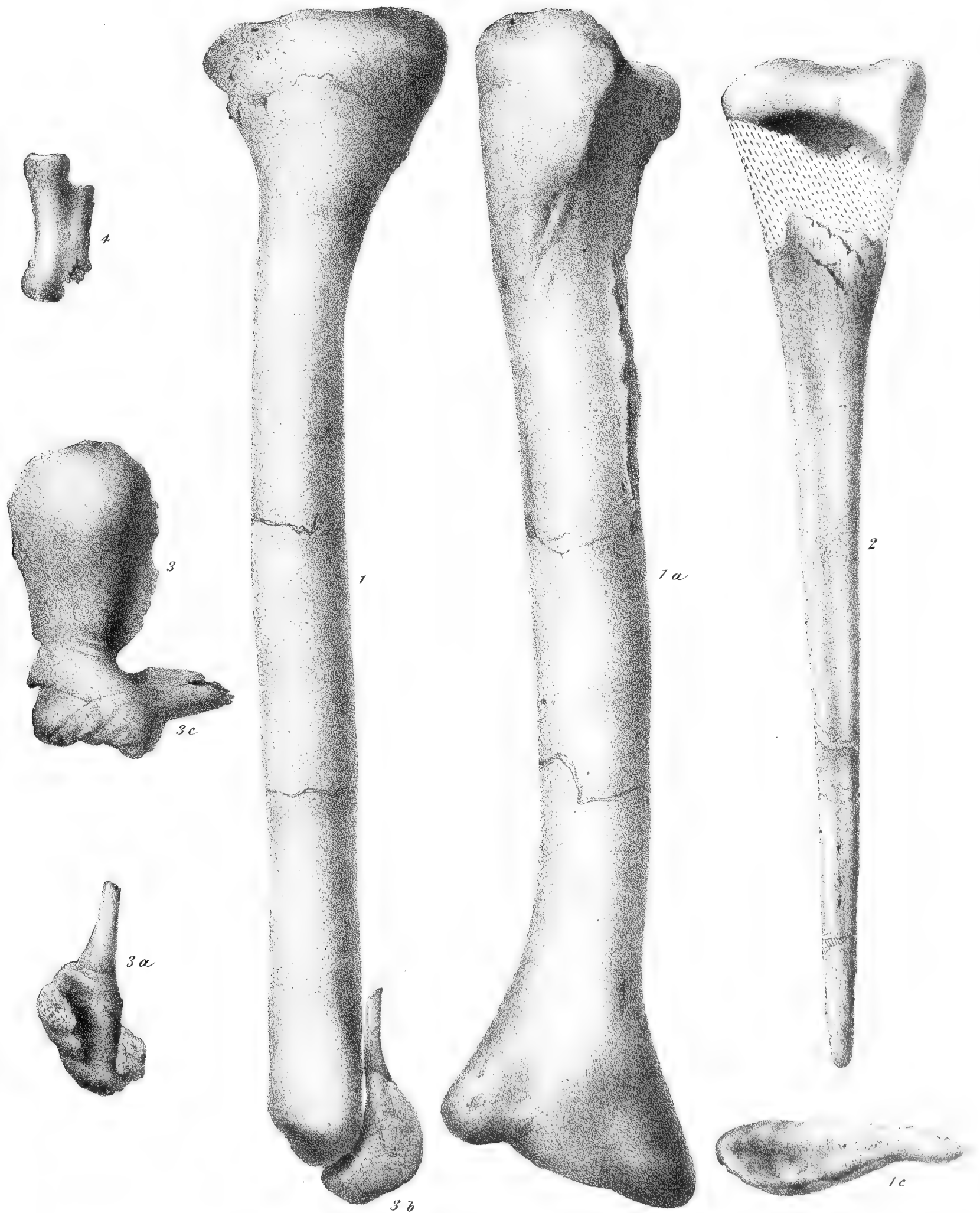
Laelaps aquilunguis.
