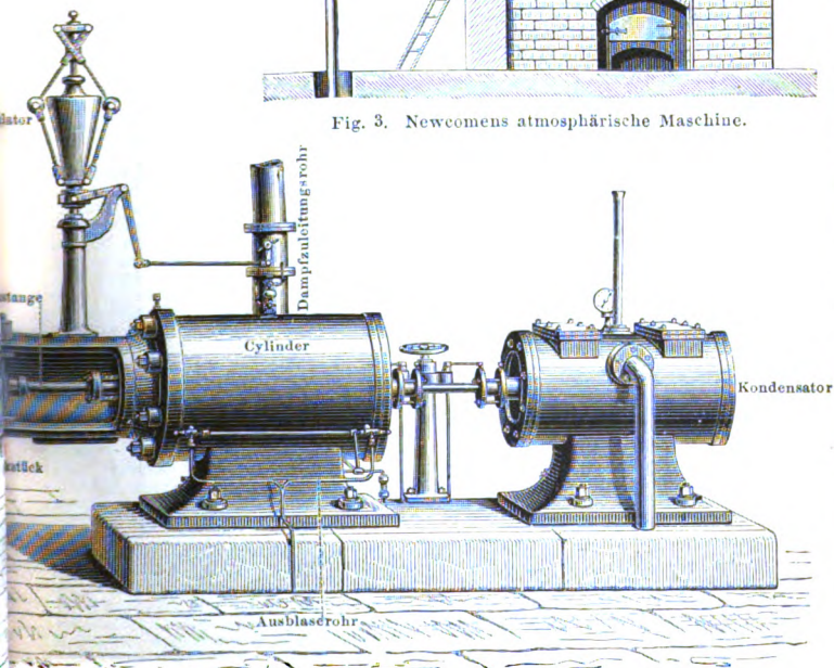
Dampfmaschine.
