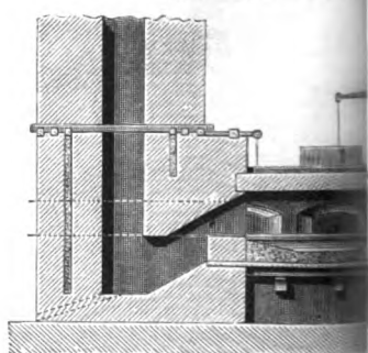
Fig. 5. Puddelofen. Län
