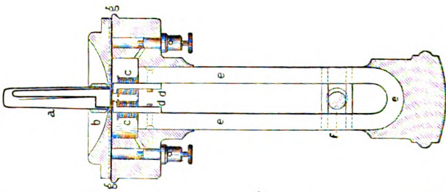
Fig. 2. Siemens' Fernsprecher (Querschnitt).
