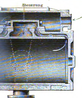
Querschnitt des Cylinders.
