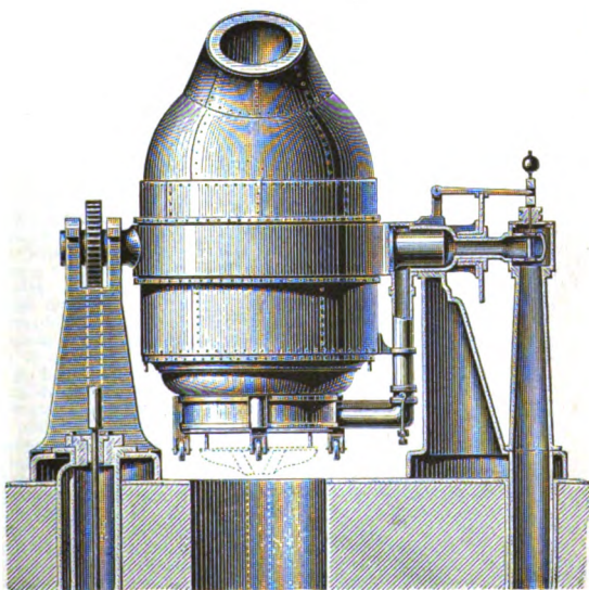
Fig. 7. Bessemerbirne.
