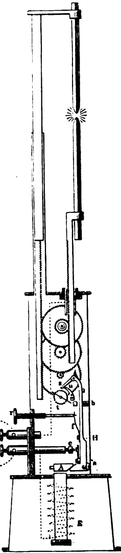
Fig. 2. Elektrische Lampe von Hefner-Alteneck (Siemens u. Halske).
