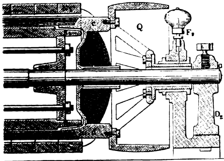
Elektrische Maschine (Durchschnitt).
