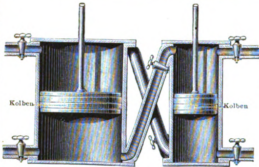
Fig. 4. Cylinder von Woolfs Expansionsmaschine.
