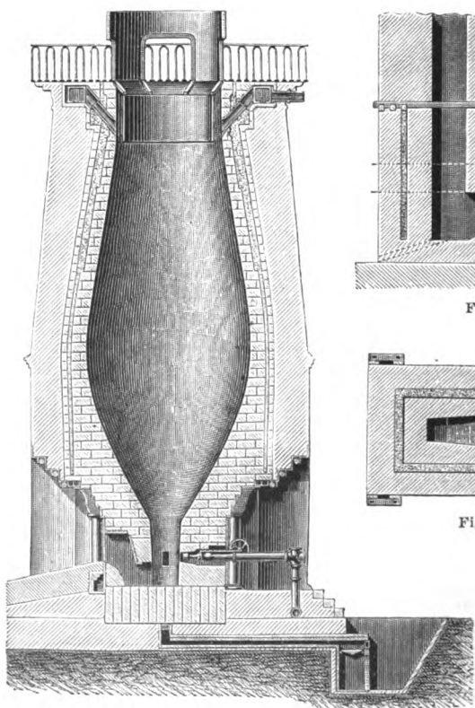
Fig. 1. Rheintischer Koks-Hochofen.
