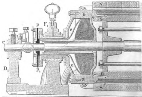
Fig. 4. Hefner-Altenecks dynamo.
