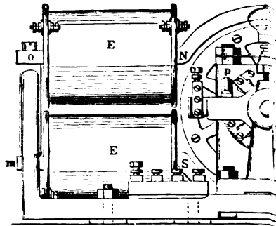
Fig. 3. Hefner-Altenecks dynamo.
