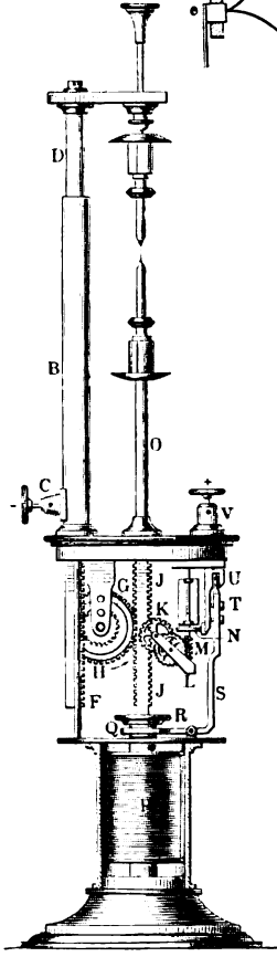
Fig. 1. Elektr. Lampe von Dubosq.
