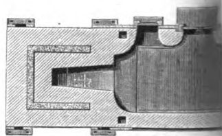
Fig. 6. Puddelofen. Quer
