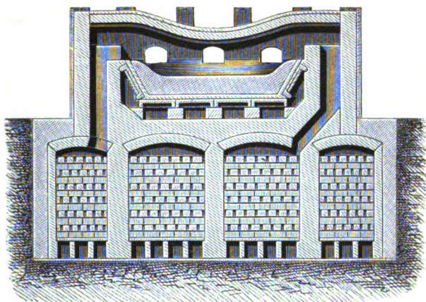
Fig. 8. Siemens-Martin-Ofen.
