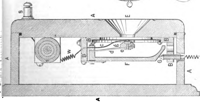
Fig. 4. Blake's Mikrophonsender.
