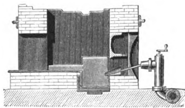
Fig. 3. Frischfeuer.
