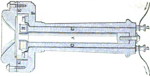
Fig. 1. Telephon von Bell.
