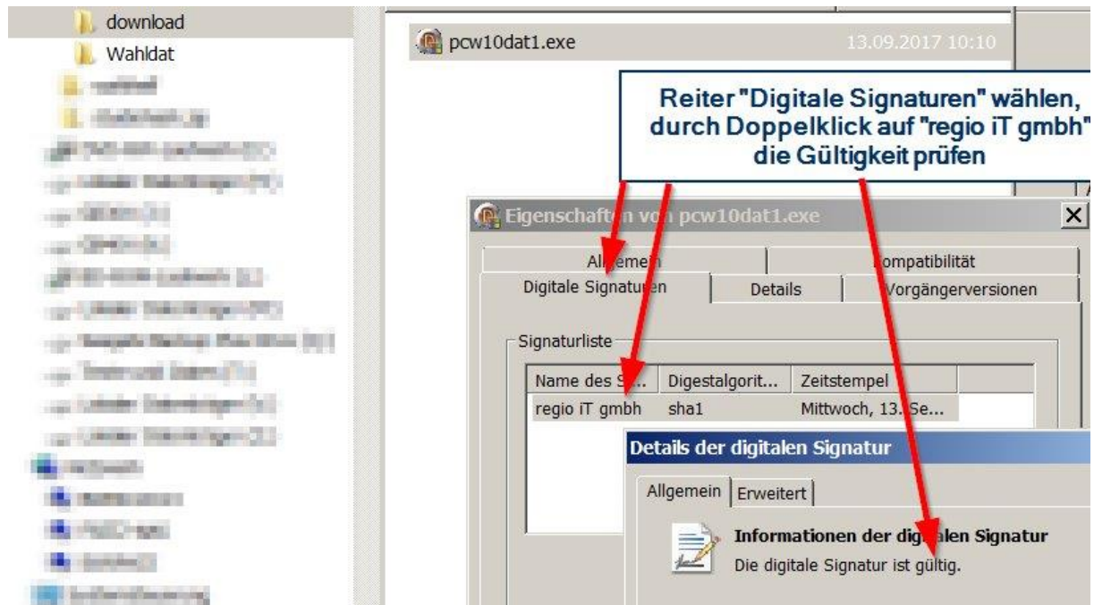
Abbildung 1. Anweisung des Herstellers zur manuellen Überprüfung der Update-Signaturen durch Nutzer
