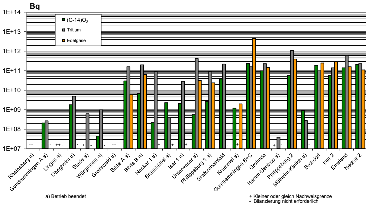
Abbildung B II 1.5-2 Ableitung radioaktiver Stoffe mit der Fortluft aus Kernkraftwerken im Jahr 2016 (C-14 als Kohlenstoffdioxid, Tritium und Edelgase) (Discharge of radioactive substances with exhaust air from nuclear power plants (C-14 as carbondioxide, tritium and noble gases) during the year 2016)
