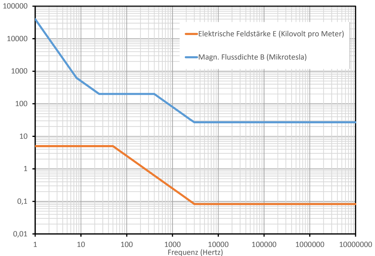
Abbildung G VI 3.1 Grenzwerte für feststehende Niederfrequenz- und Gleichstromanlagen (26. BImSchV) (Limit values for fixed low-frequency and DC installations - 26 th BImSchV)
