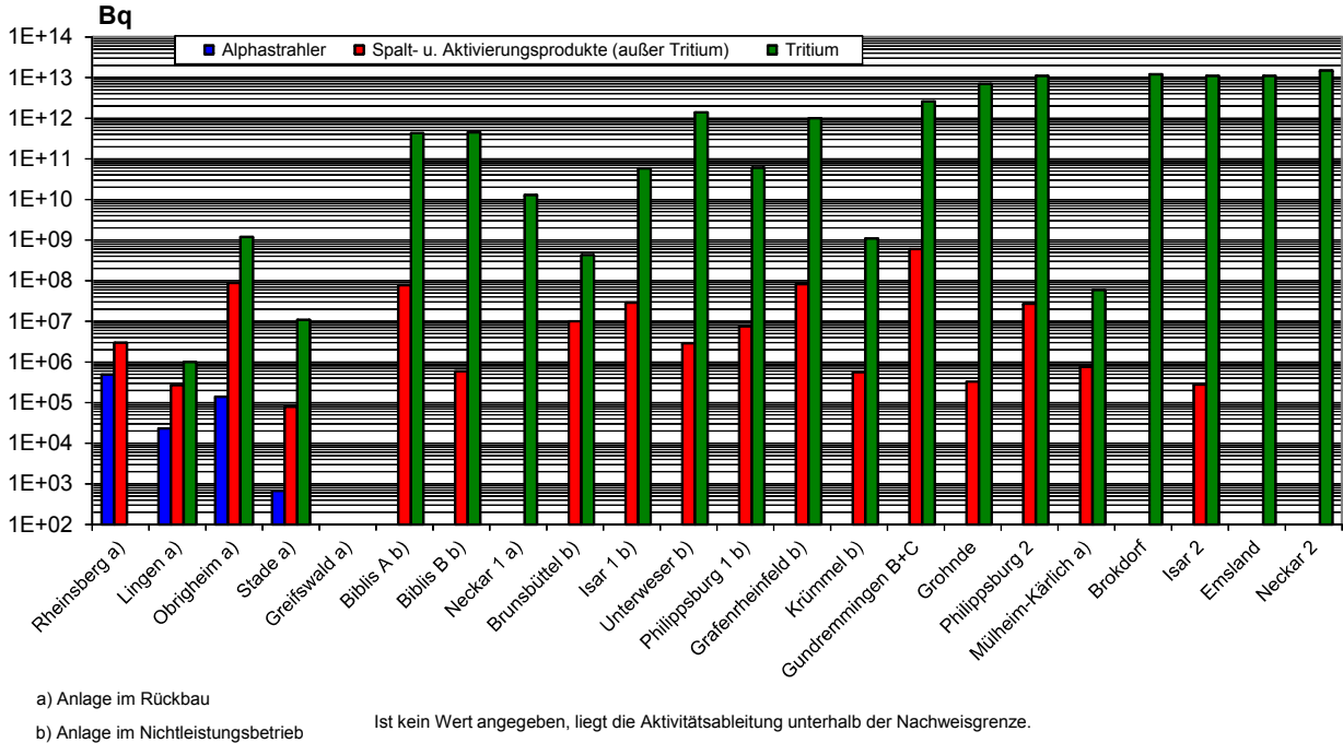
Abbildung B II 1.5-5 Ableitung radioaktiver Stoffe mit dem Abwasser aus Kernkraftwerken im Jahr 2016 (Alphastrahler, Summenwerte und Tritium) (Discharges of radioactive substances with waste water from nuclear power plants in the year 2016 (alpha sources, summation values, and tritium))
