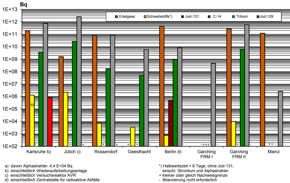
Abbildung B II 1.5-3 Ableitung radioaktiver Stoffe mit der Fortluft aus Forschungszentren im Jahr 2016 (Schwebstoffe, I-131 und I-129, C-14 (gesamt), Tritium und Edelgase)
