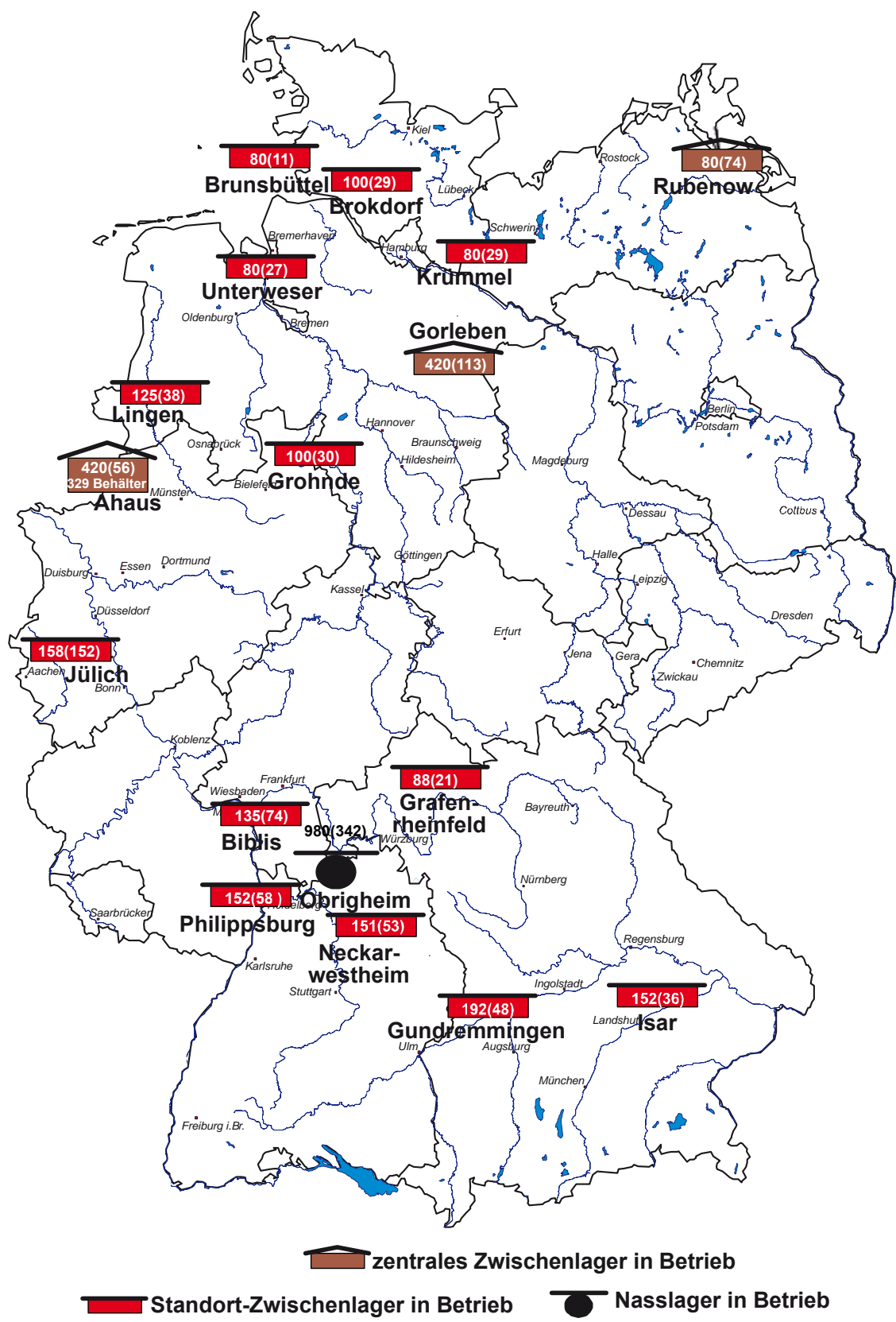
Abbildung B II 1.4-1 Zwischenlager für bestrahlte Brennelemente in Deutschland im Jahr 2016 mit Anzahl der Stellplätze (Belegung in Klammern, Stand 31.12.2016) bzw. beim Nasslager Obrigheim Positionen für Brennelemente
