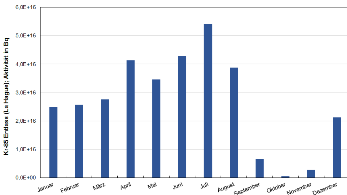
Abbildung B II 2.1-3 Monatlicher Kr-85-Entlass der Wiederaufbereitungsanlage La Hague für das Jahr 2016 ( Monthly emission of Kr-85 from La Hague reprocessing plant in 2016 )
