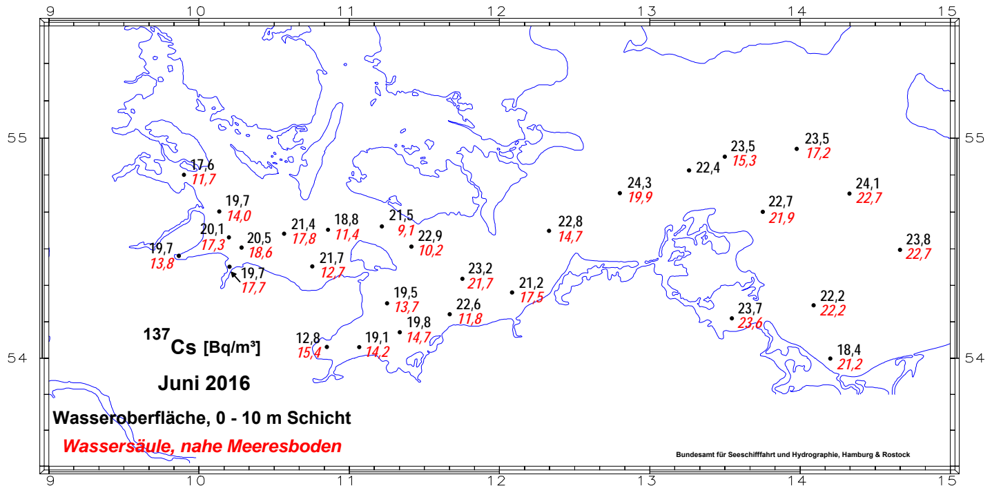
Abbildung B II 2.2-3 Verteilung der Aktivitätskonzentration von Cs-137 (Bq/m 3 ) im Oberflächen- und Bodenwasser der westlichen Ostsee im Juni 2016 (Spatial distribution of the activity concentration of Cs-137 (Bq/m 3 ) in surface and bottom sea water of the western Baltic Sea in June 2016)
