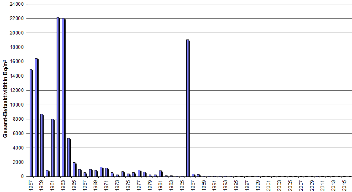
Abbildung B II 2.1-10 Dem Erdboden durch Niederschläge zugeführte langlebige Gesamt-β-Aktivität - Jahresmittelwerte der Jahressummen an den DWD-Messstationen von 1957 bis 2016 ( Deposition of additional long-lived total β-activity due to precipitation - Annual mean value for the total annual levels determined at the DWD measuring stations, 1957 - 2016 )
