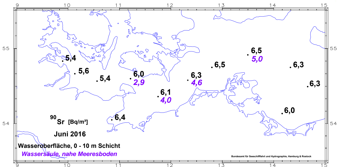
Abbildung B II 2.2-4 Verteilung der Aktivitätskonzentration von Sr-90 (Bq/m 3 ) im Oberflächen- und Bodenwasser der westlichen Ostsee im Juni 2016
