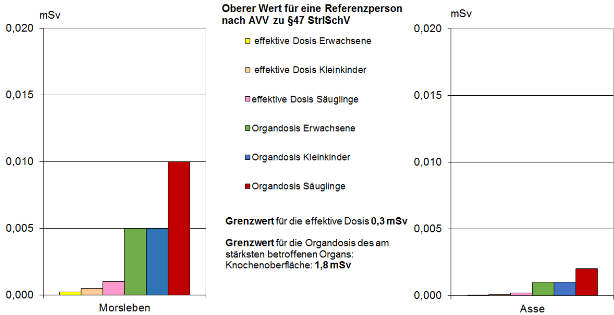
Abbildung B II 1.6-4 Strahlenexposition in der Umgebung des Endlagers Morsleben und der Schachtanlage Asse durch die Ableitung radioaktiver Stoffe mit der Fortluft im Jahr 2016 (Radiation exposure in the surroundings of the final repositories due to the discharge of radioactive substances with exhaust air in 2016)
