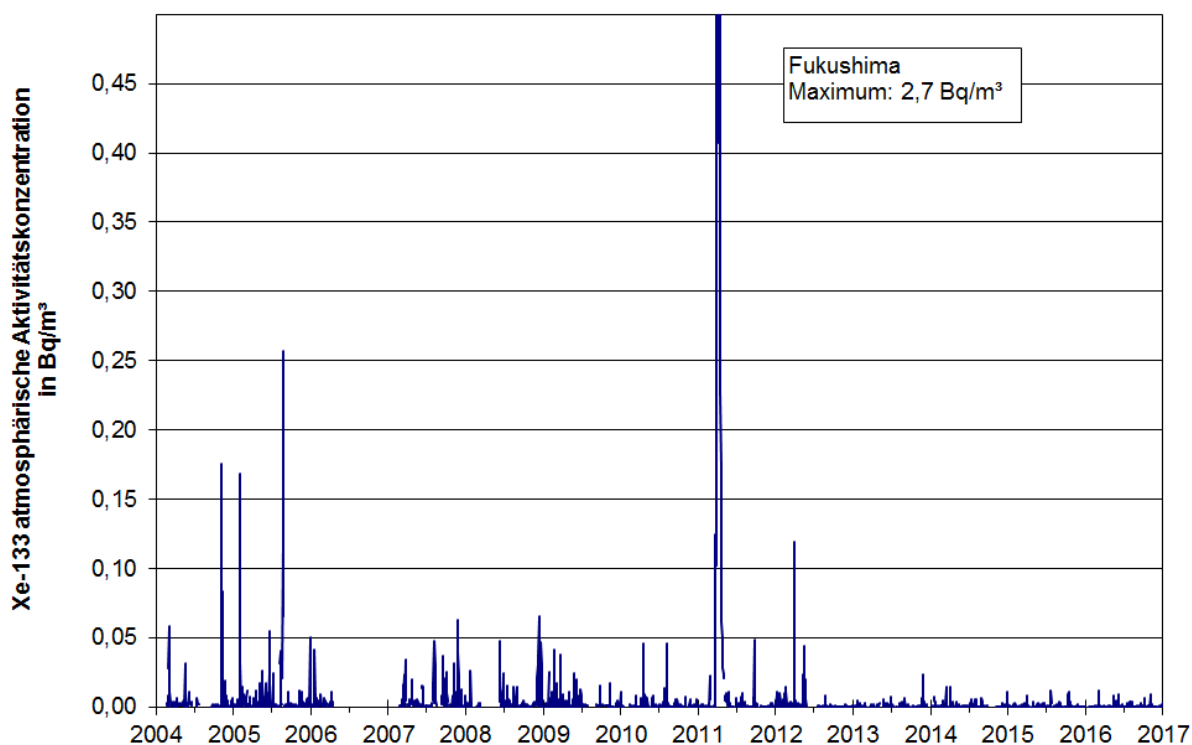
Abbildung B II 1.2-1 Zeitreihe der Xe-133-Aktivitätskonzentration in den Jahren 2004 bis 2016 an der CTBT-Station RN33 auf dem Schauinsland (Time series of Xe-133-activity concentration at CTBT-station RN33 at Schauinsland mountain for the years 2004 to 2016)
