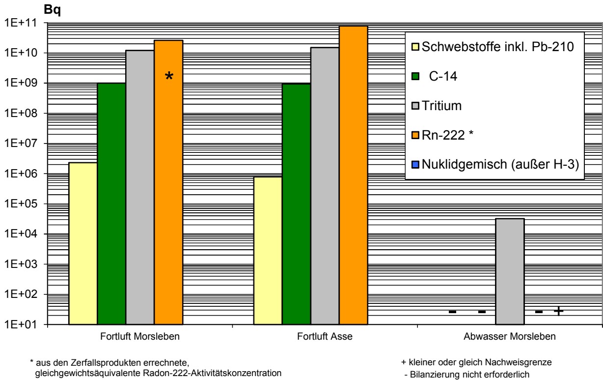
Abbildung B II 1.5-4 Ableitung radioaktiver Stoffe mit der Fortluft und dem Abwasser aus dem Endlager Morsleben und der Schachanlage Asse im Jahr 2016 (Discharges of radioactive substances with exhaust air and waste water from the Asse mine and the radioactive waste repository Morsleben in 2016)
