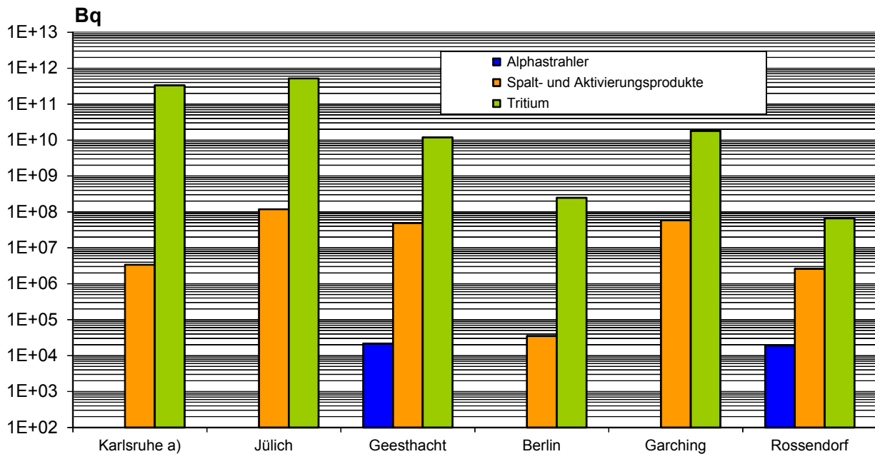
Abbildung B II 1.5-6 Ableitung radioaktiver Stoffe mit dem Abwasser aus Forschungszentren im Jahr 2016 (Alphastrahler, Summenwerte und Tritium) (Discharges of radioactive substances with waste water from research centres in the year 2016 (alpha sources, summation values, and tritium))
