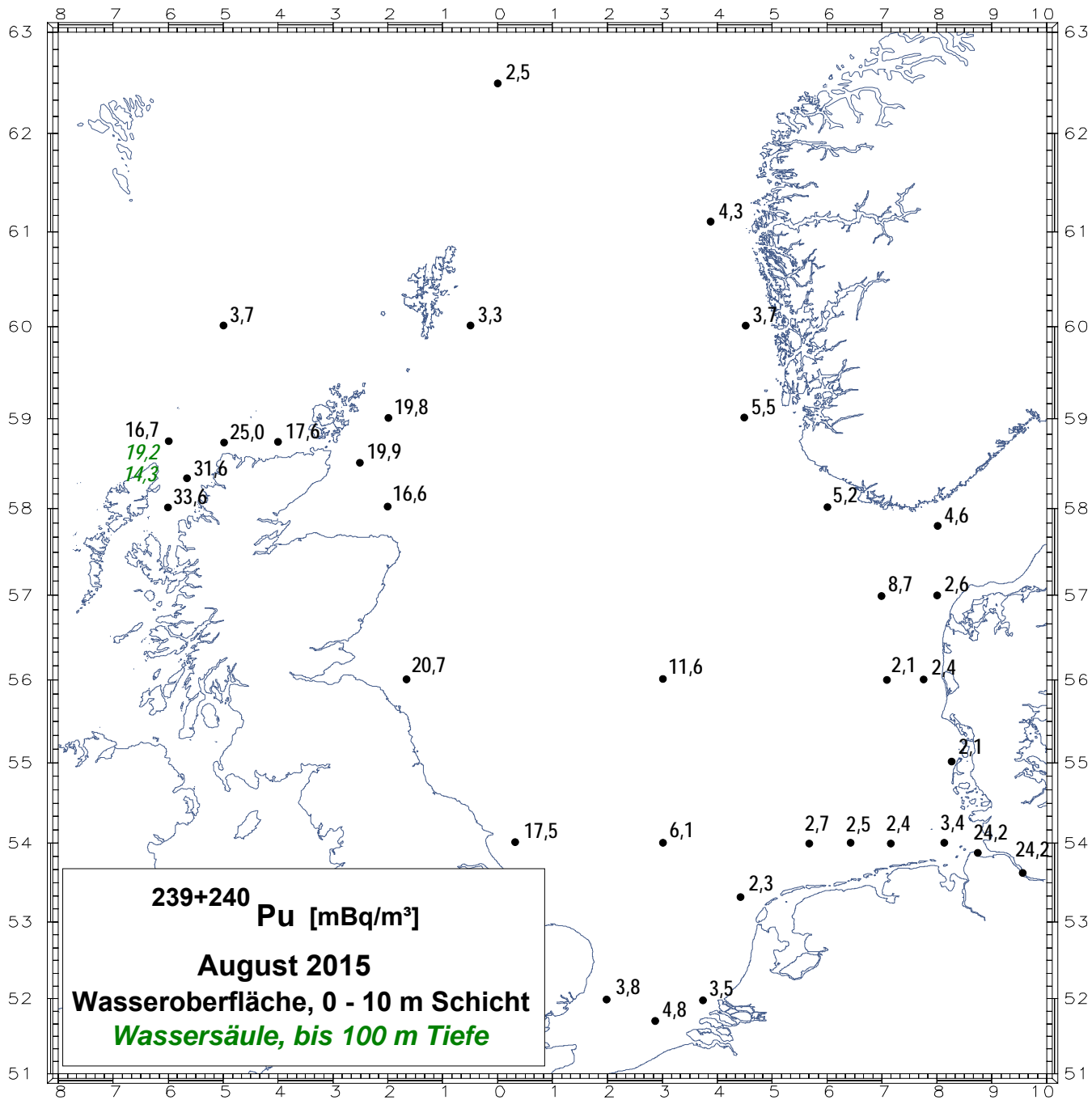
Abbildung B II 2.2-2 Die Verteilung der Aktivitätskonzentration von Pu-(239+240) ( Bq/m^3 ) im Wasser der Nordsee im August 2015 (Distribution of the activity concentration of Pu-(239+240) ( Bq/m^3 ) in seawater of the North Sea in August 2015)
