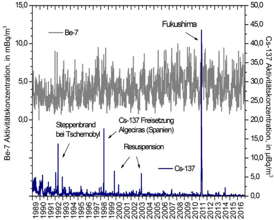
Abbildung B II 2.1-5 Aktivitätskonzentration von Cs-137 und Be-7 in der bodennahen Luft am Probenentnahmeort Schauinsland (Activity concentration of Cs-137 and Be-7 in ground level air at Schauinsland measuring station)
