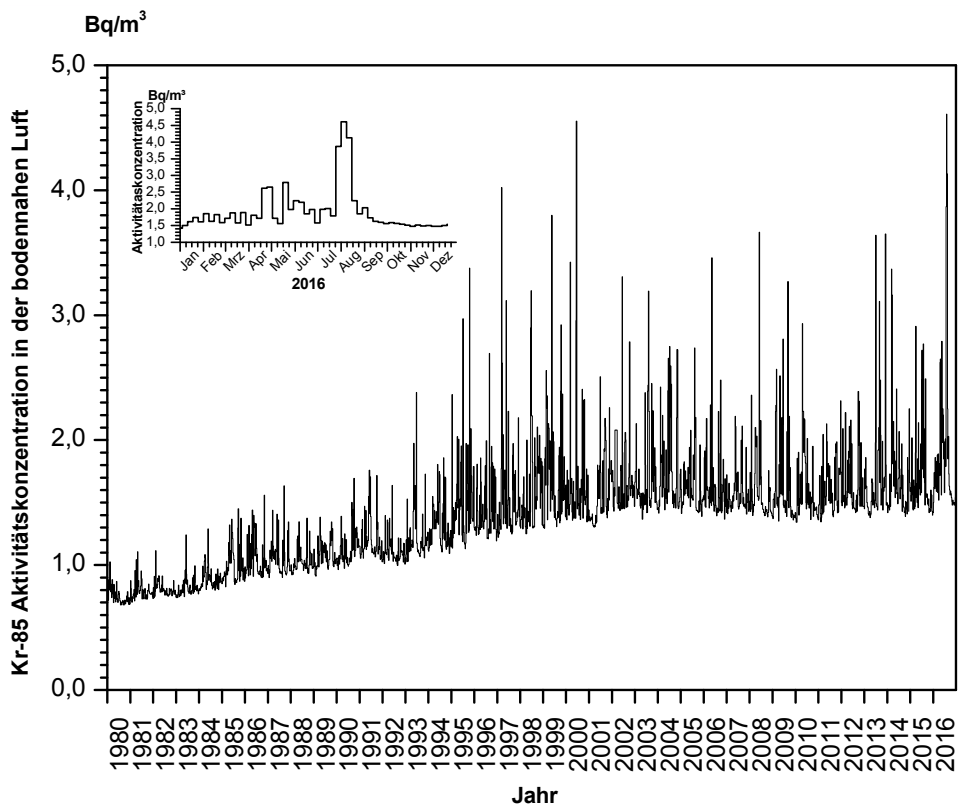
Abbildung B II 2.1-2 Kr-85-Aktivitätskonzentration in der bodennahen Luft am Probenentnahmeort Schauinsland (Kr-85-activity concentration in air close to ground level at the sampling location Freiburg/Schauinsland)
