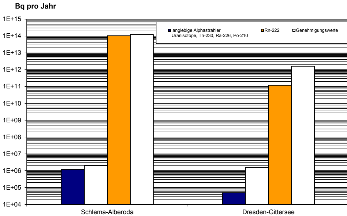
Abbildung B I 2.1-1 Ableitung radioaktiver Stoffe mit den Abwettern bzw. der Fortluft in die Atmosphäre aus den Wismut-Sanierungsgebieten im Jahr 2016 (Discharge of radioactive substances into the atmosphere with exhaust air in the Wismut remediation areas 2016)
