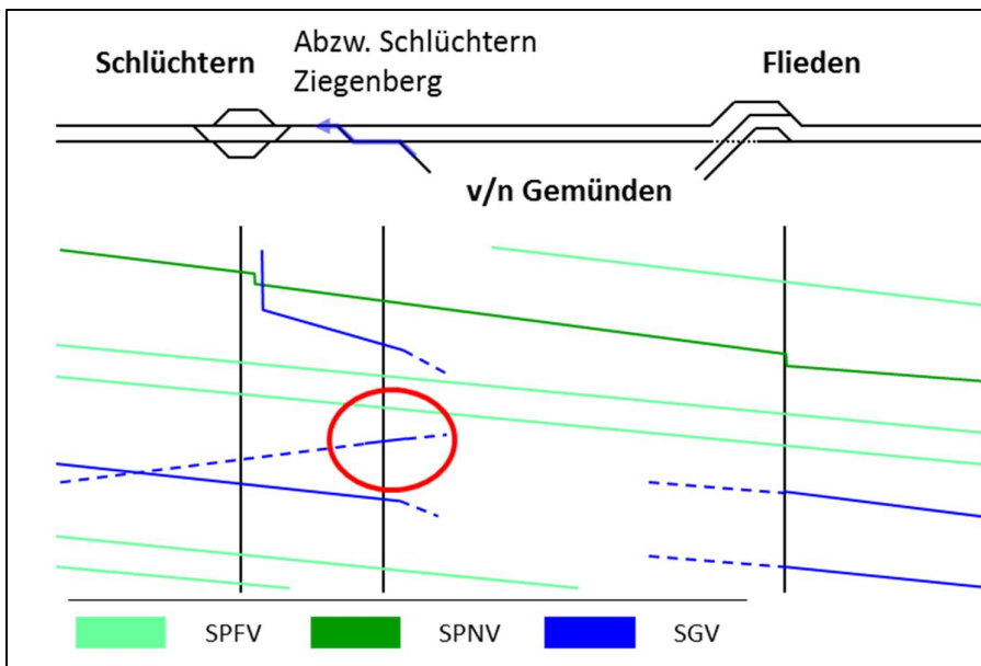
Abbildung 9: Engpass Schlüchtern Ziegenberg mit höhengleich einfädlerndem SGV
