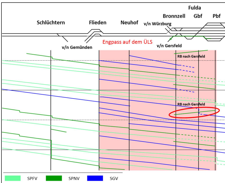
Abbildung 12: Engpass Flieden - Fulda
