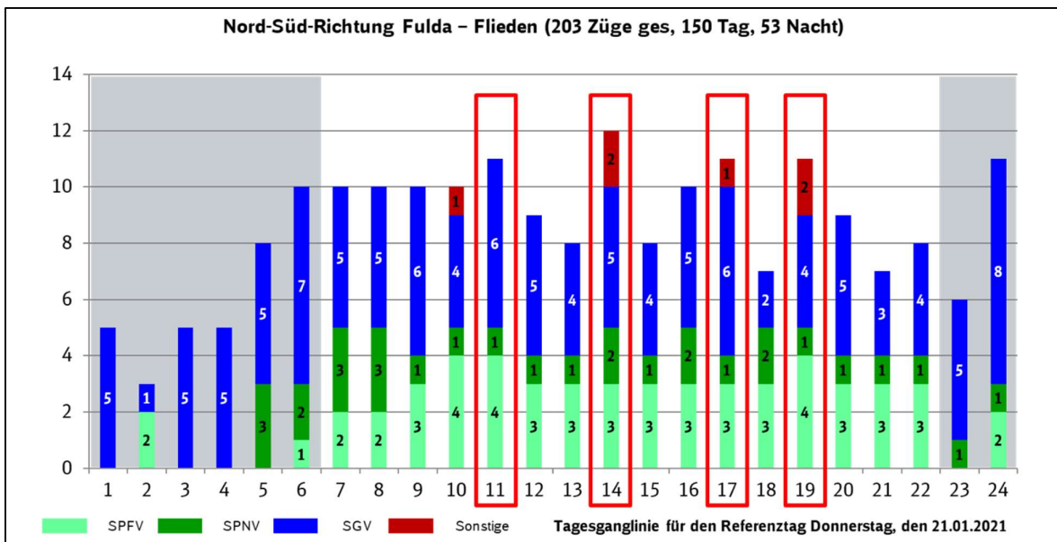
Abbildung 6: Tagesganglinie für Donnerstag 21.01.2021 - von Fulda nach Flieden
