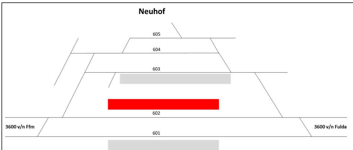
Abbildung 17: Zusätzlicher Bahnsteig im Bahnhof Neuhof an Gleis 602
