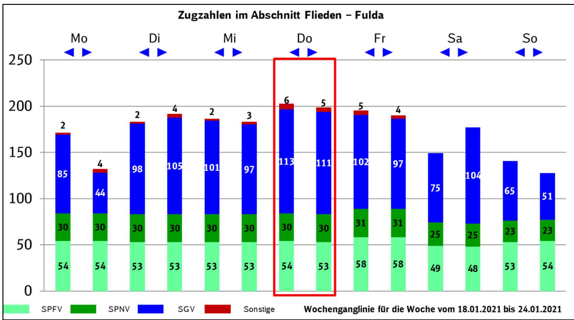
Abbildung 4: Wochenganglinie 18.01.2021 bis 24.01.2021 im Abschnitt Flieden - Fulda
