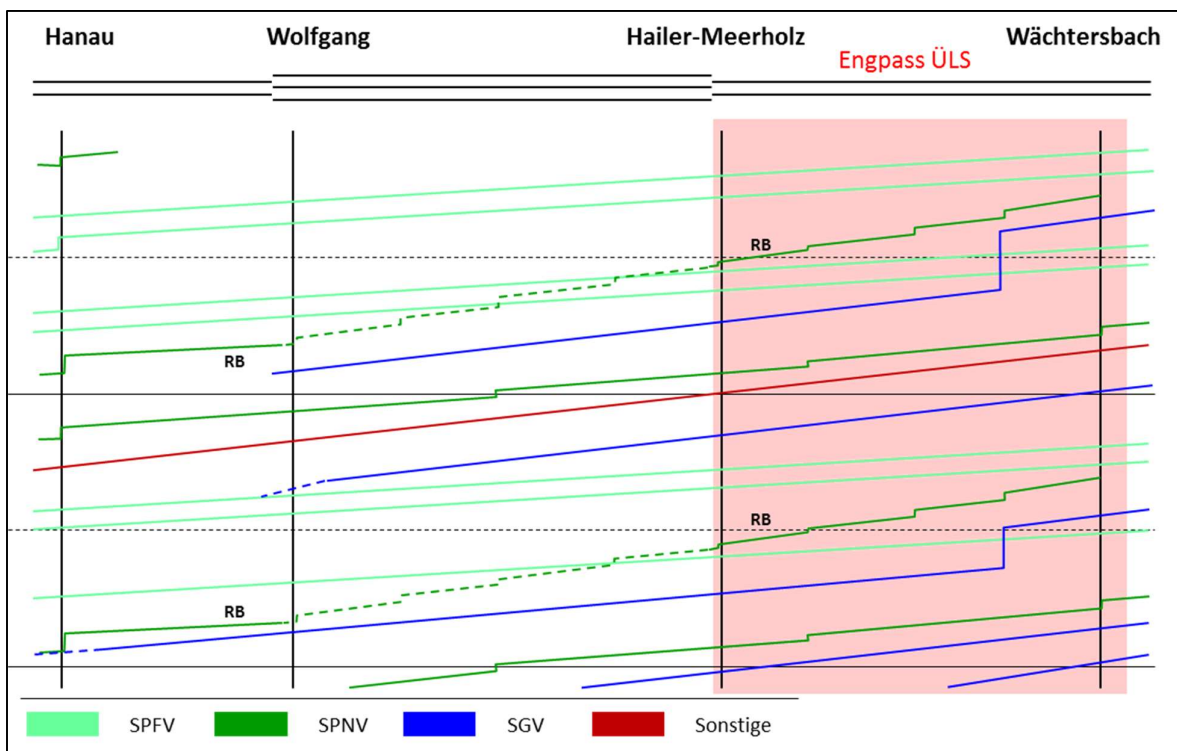
Abbildung 8: Engpass Hailer-Meerholz - Wächtersbach
