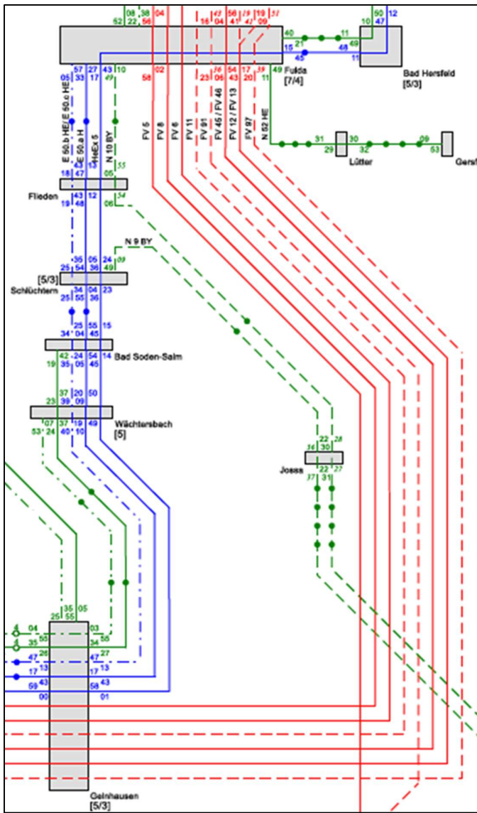
Abbildung 14: Zielfahrplan Deutschland-Takt
