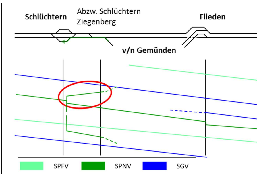
Abbildung 10: Engpass Schlüchtern Ziegenberg mit Gegengleisfahrt der RB 53
