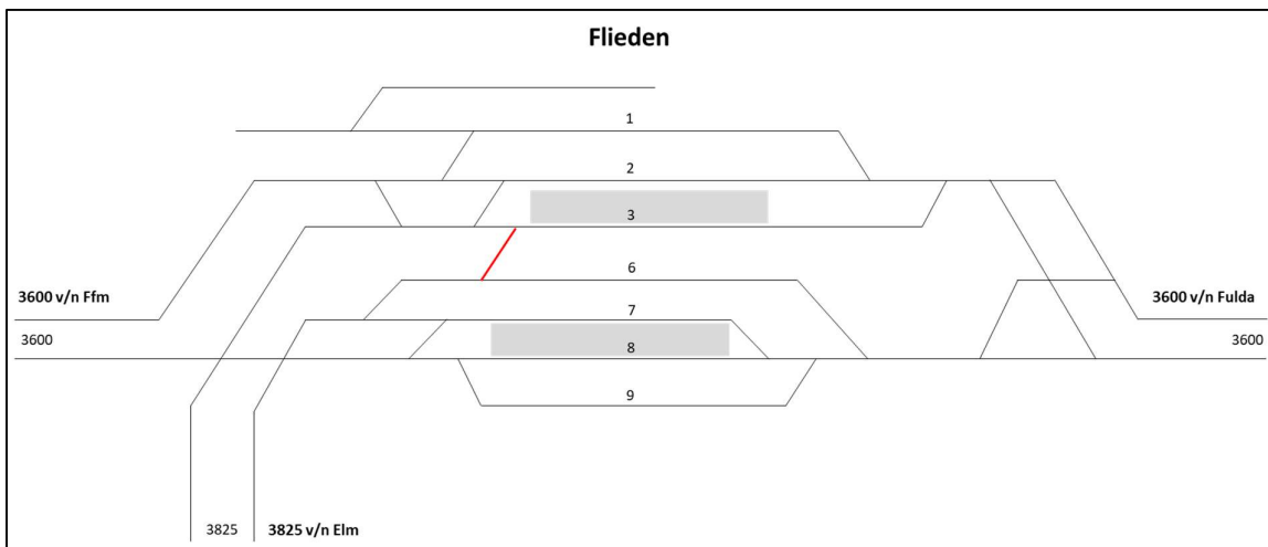
Abbildung 19: Zusätzliche Weichenverbindung zum Wenden der RB 53
