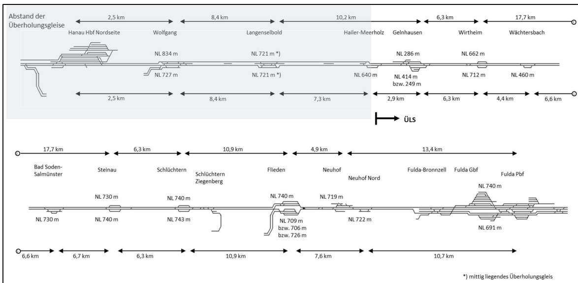
Abbildung 2: Infrastrukturübersicht des Abschnittes Hanau - Fulda
