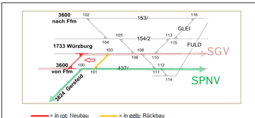
Abbildung 20: Verschiebung der Weichenverbindung in Fulda-Bronnzell
