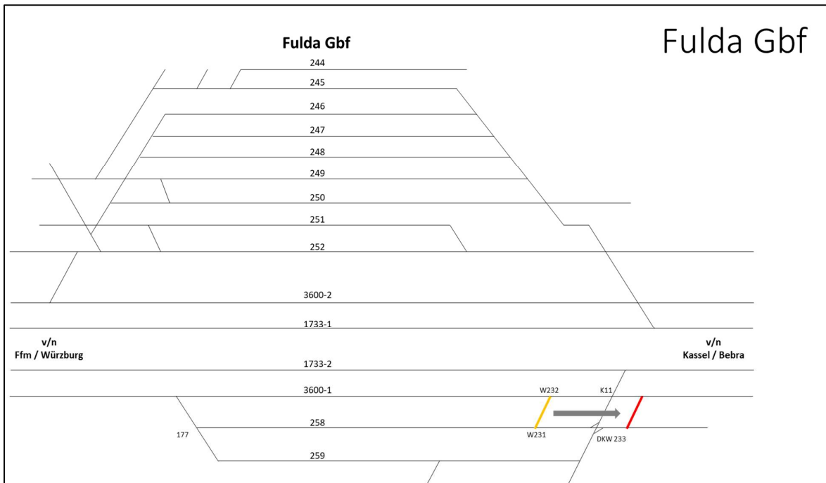
Abbildung 22: Verlängerung Gleis 258 durch Weichenverschiebung
