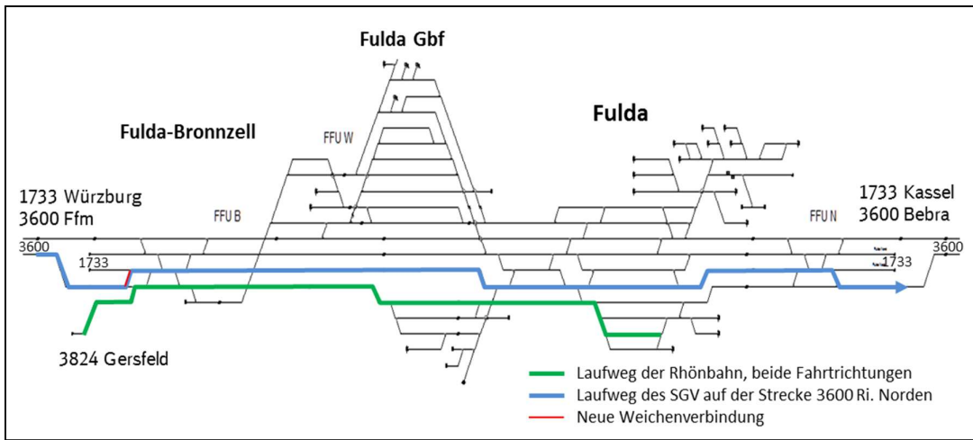
Abbildung 21: Parallele Fahrmöglichkeiten durch Infrastrukturanpassung in Fulda-Bronzell
