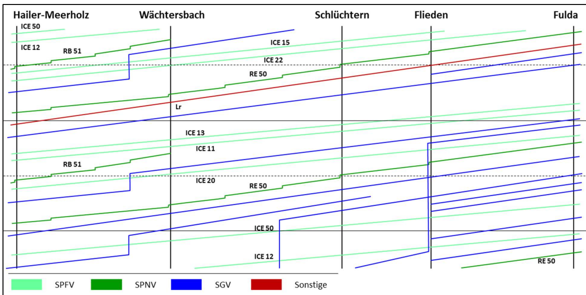
Abbildung 7: Fahrplanstruktur des Mischverkehrs zwischen Hailer-Meerholz und Fulda
