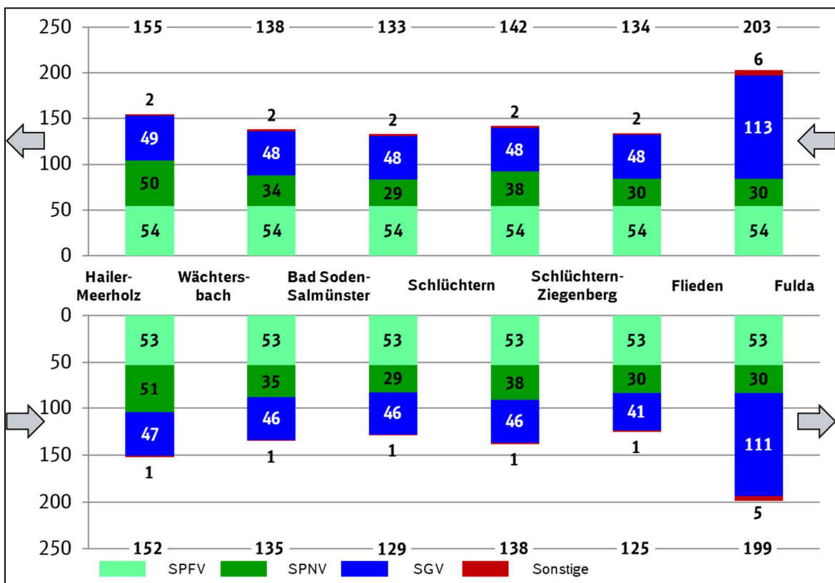
Abbildung 3: Abschnittsbezogene Zugzahlen nach Verkehrsarten am 21.01.2021
