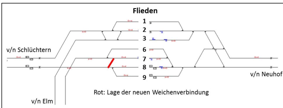
Abbildung 18: Infrastrukturanpassung im Rahmen des ESTW Flieden
