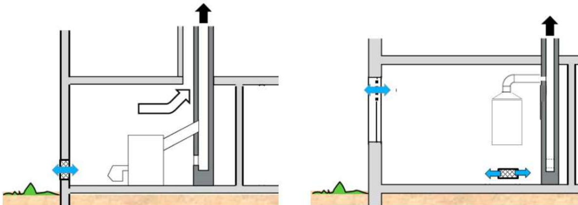
Abb. 52 Lüftungsöffnung
