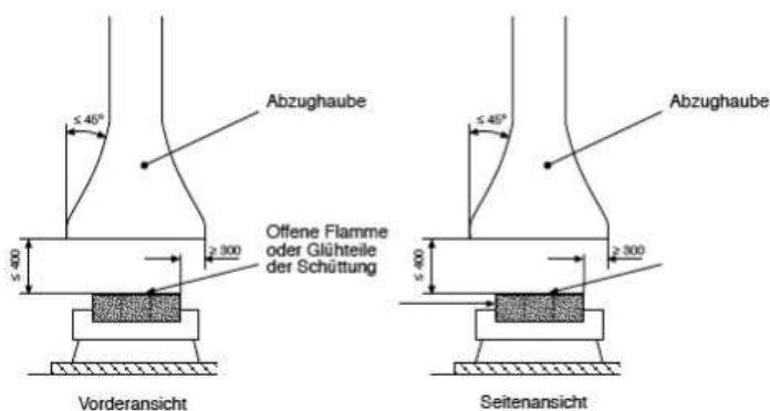
Abb. 86 Massvorgaben an freihängende Abzugshaube an das Gerät angeschlossen
