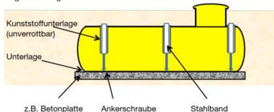
Abb. 5 Auftriebssicherung
