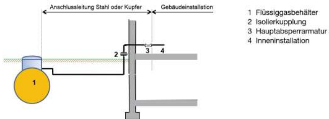
Abb. 23 Anschluss überflur
