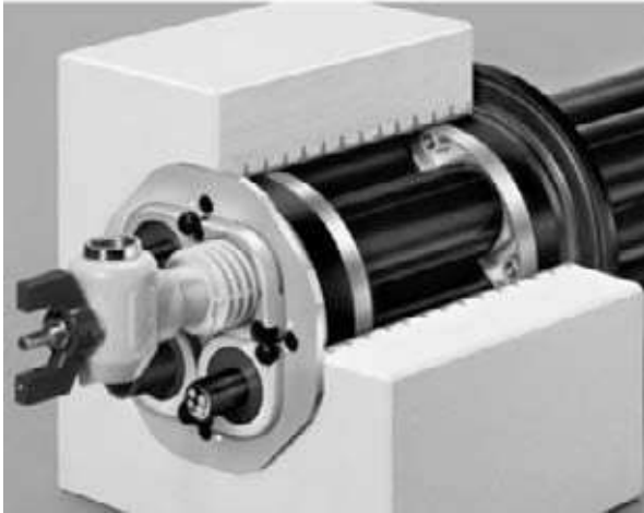
Abb. 22 Mehrsparten-Gebäudeeinführungskombination
