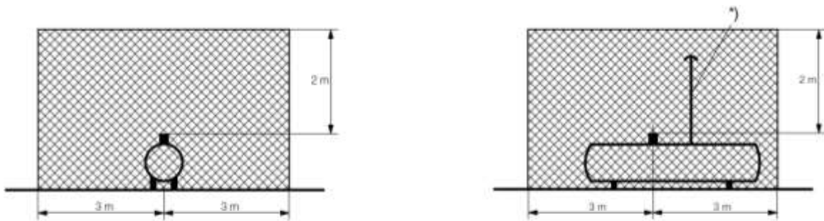
Abb. 11 Füllstutzen am Behälter (Peilrohr, Füllstandsanzeiger, usw.)
