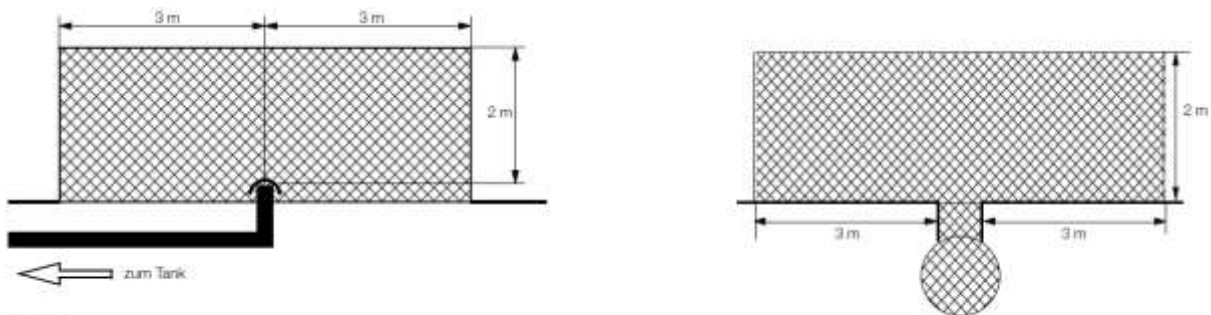
Abb. 12 Füllstutzen an Füllleitung (im Gelände) und Füllstutzen zu erdgedecktem Behälter
