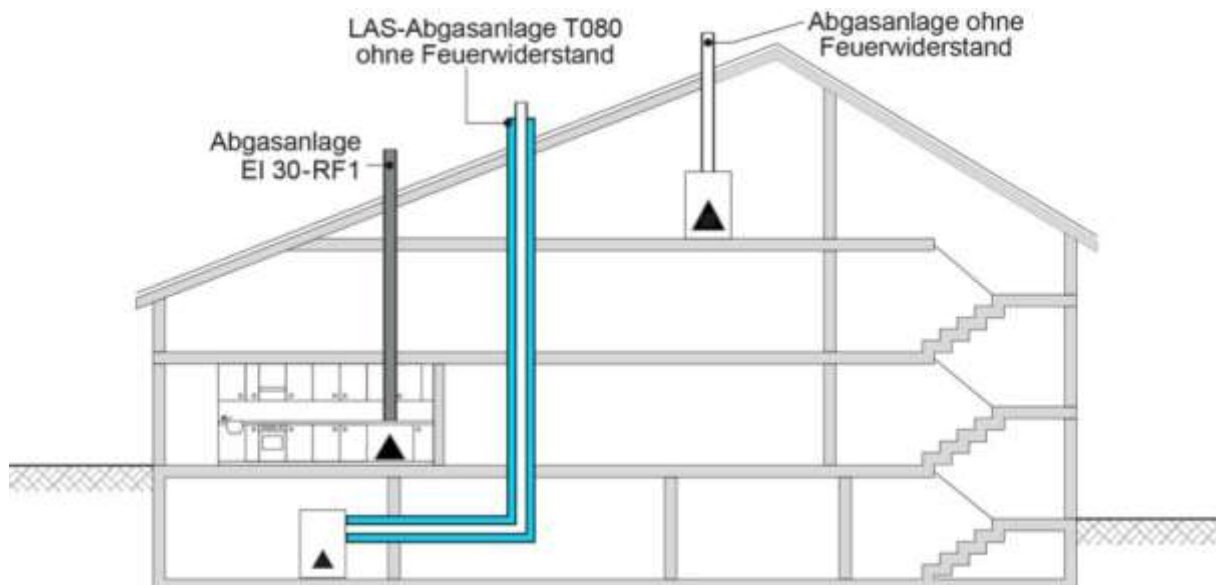
Abb. 78 Beispiel Einfamilienhäuser und Gebäude mit geringen Abmessungen
