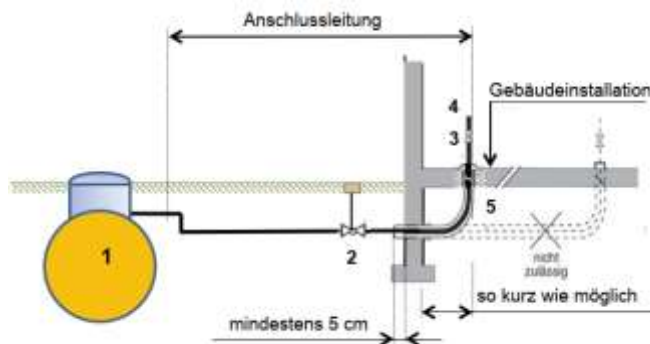
Abb. 26 Anschluss unterflur mit flexibler Hauseinführung in ein nicht unterkellertes Gebäude
