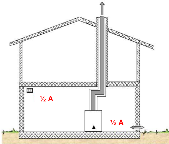
Abb. 55 Überfluranlage (über 70 kW)
