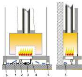
Cheminéeanlage mit Frischluft aus dem Aufstellraum
