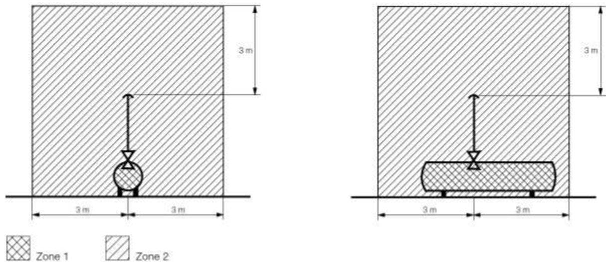
Abb. 14 Flüssiggasbehälter im Freien mit Sicherheitsabblaseventil und Abblaseleitung
