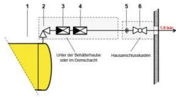
Variante B: Mit Druckbegrenzer Verteildruck 1,5 bar
