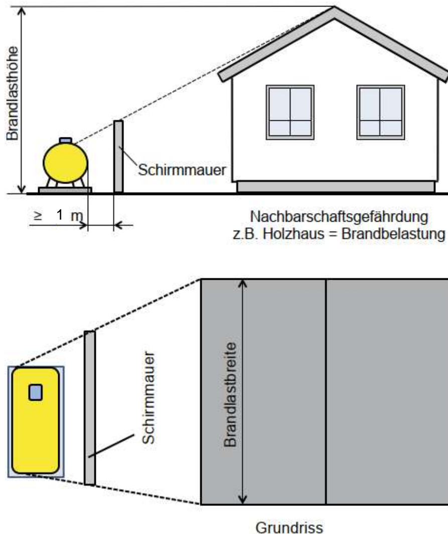
Abb. 8 Schirmmauer zwischen Flüssiggasbehälter und Gebäude
