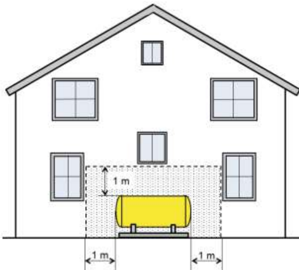
Abb. 7 Zusätzliche Schutzabstände
