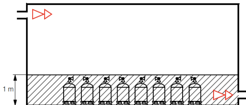
Abb. 13 Flüssiggaslagerraum mit natürlicher oder künstlicher Luft
