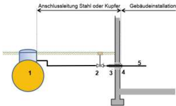
Abb. 25 Anschluss unterflur mit Ausziehsicherung
