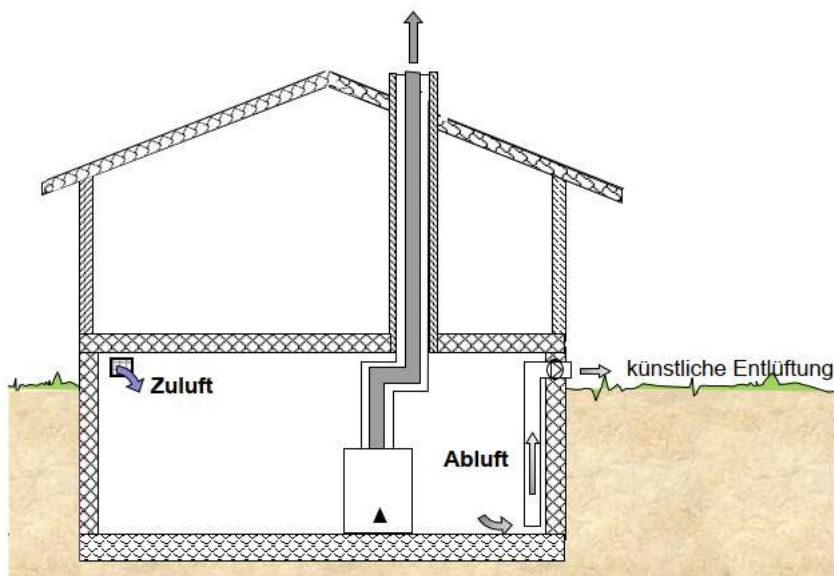
Abb. 56 Unterfluranlage über 70 kW
