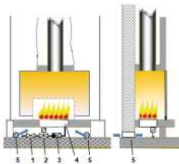
Cheminéeanlage an Aussenwand mit Frischluftzufuhr
