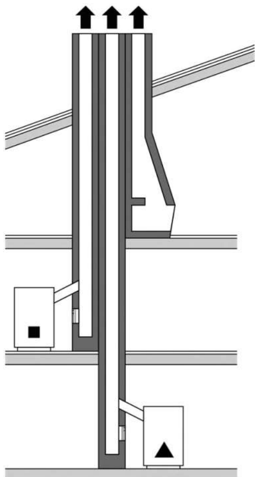
Abb. 62 Anschlüsse an separate Abgasanlagen
