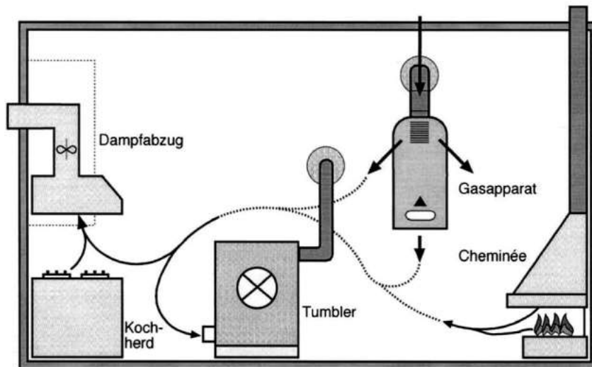
Abb. 51 Beeinträchtigung der Verbrennungsluftzufuhr
