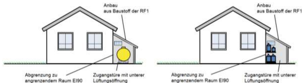
Abb. 10 Flüssiggaslager im separaten Anbau
