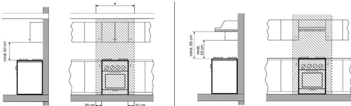
Abb. 45 KÜcheneinbauten
