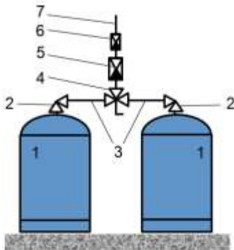
Abb. 20 2er-Flaschenrampe
