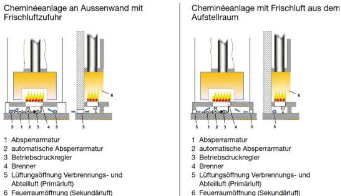
Abb. 82 Cheminéeanlagen mit offenem Feuerraum (SN EN 509)
