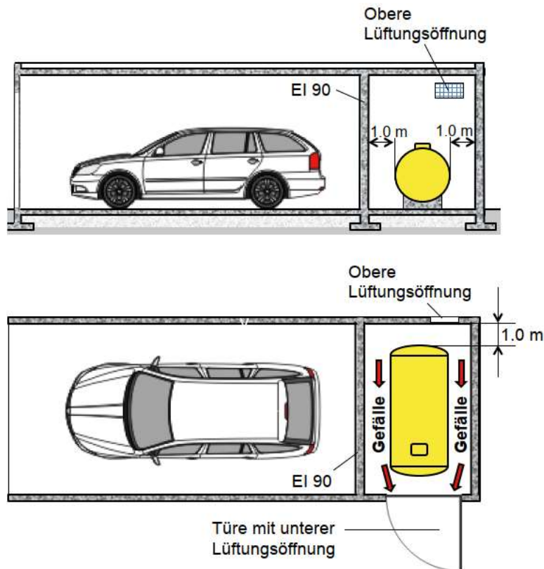
Abb. 9 Flüssiggasanlagen in Räumen
