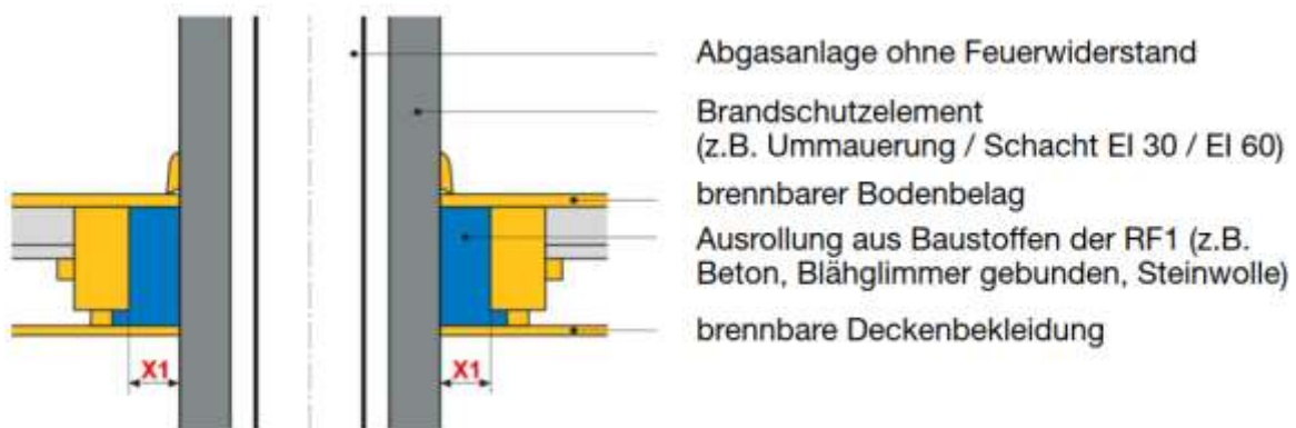
Abb. 70 Durchführung durch Holzdecke - Abgasanlage ohne Feuerwiderstand
