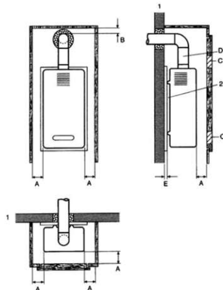
Abb. 44 Gasverbrauchsapparat in Schränken und Schrankküchen
