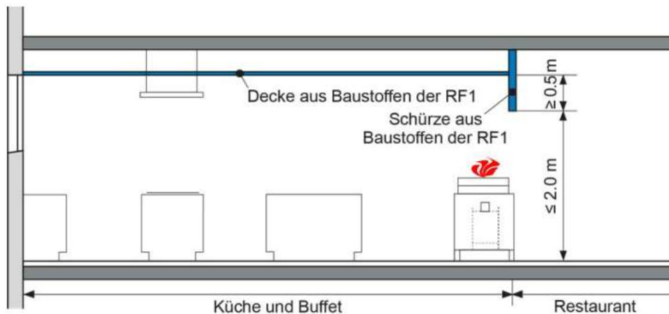
Abb. 47 Küche und Buffet mit Koch- und Grillapparat / Pizzaofen
