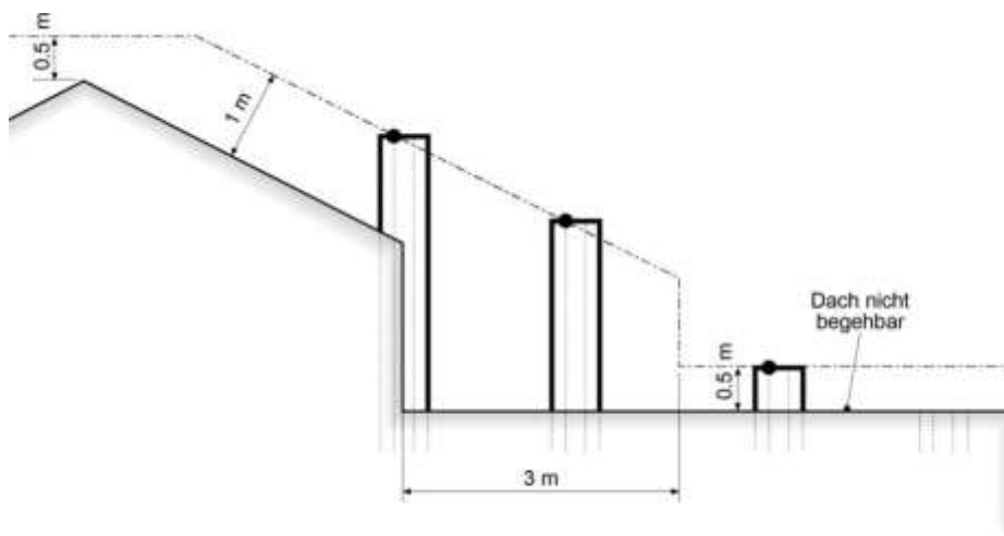
Abb. 65 Beispiel Anbauten
