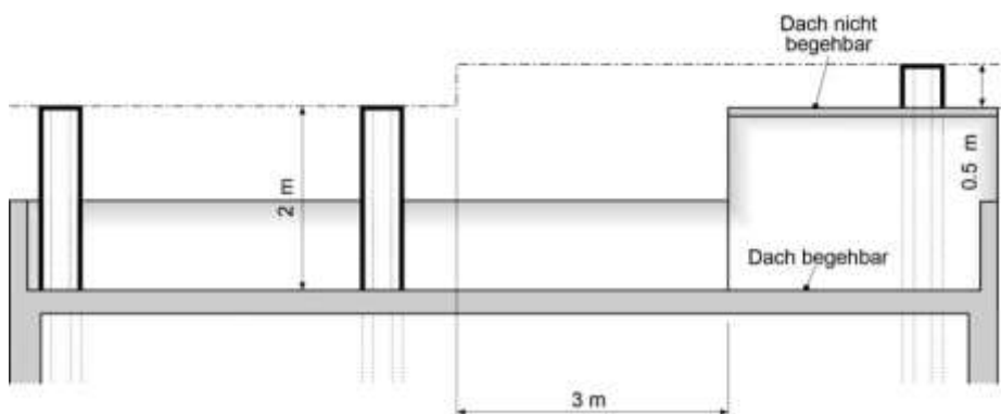
Abb. 66 Beispiel Flachdächer
