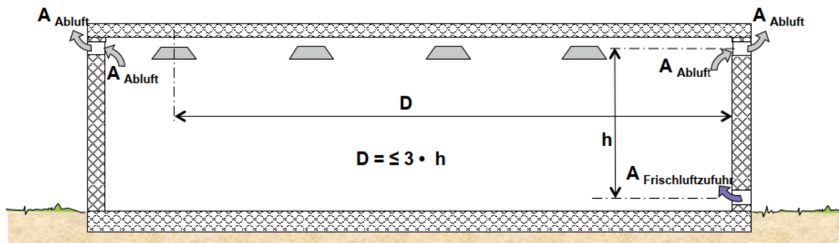
Abb. 88 Abluftöffnung in der Aussenwand
