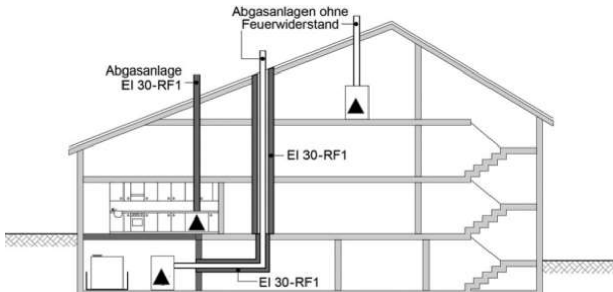
Abb. 76 Beispiel Einfamilienhäuser
