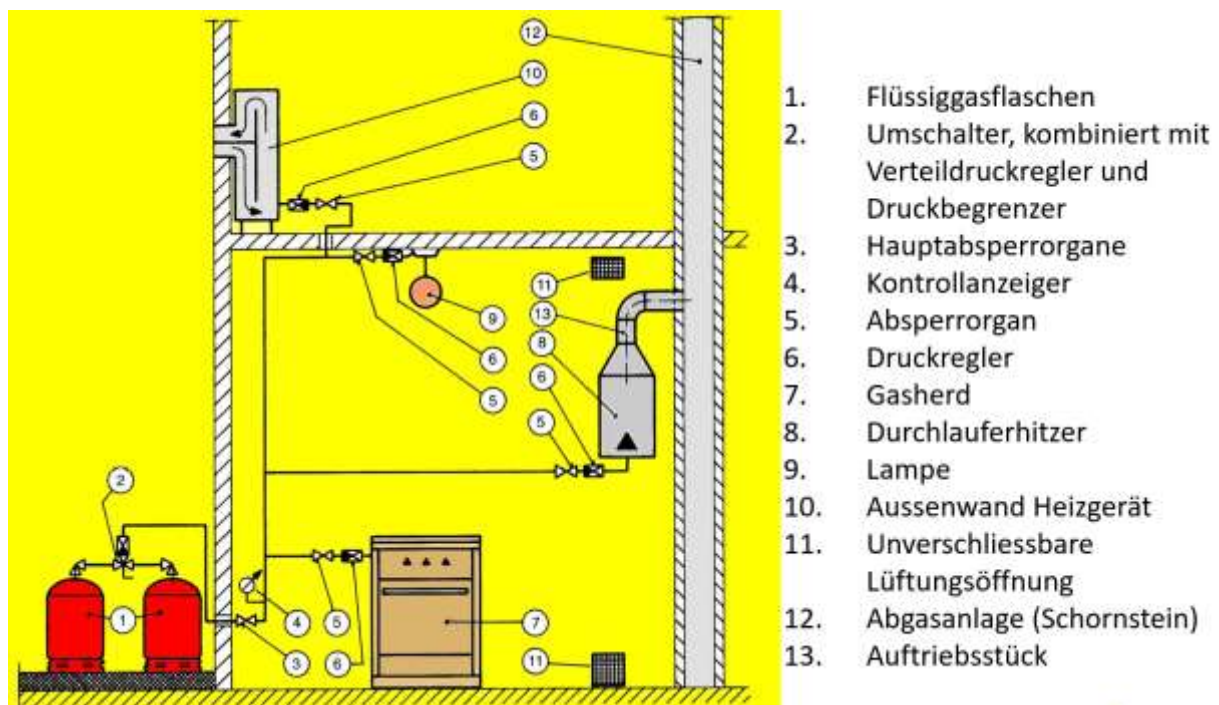
Abb. 33 Flüssiggasinstallationen im Haushalt (Prinzip Schema)
