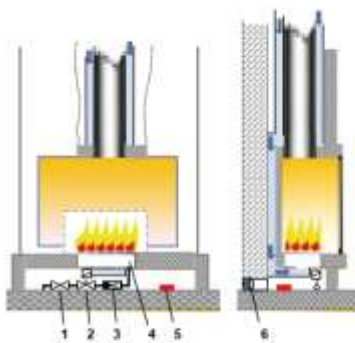
Cheminéeanlage mit LAS, Gaswarnanlage und künstliche Lüftung
