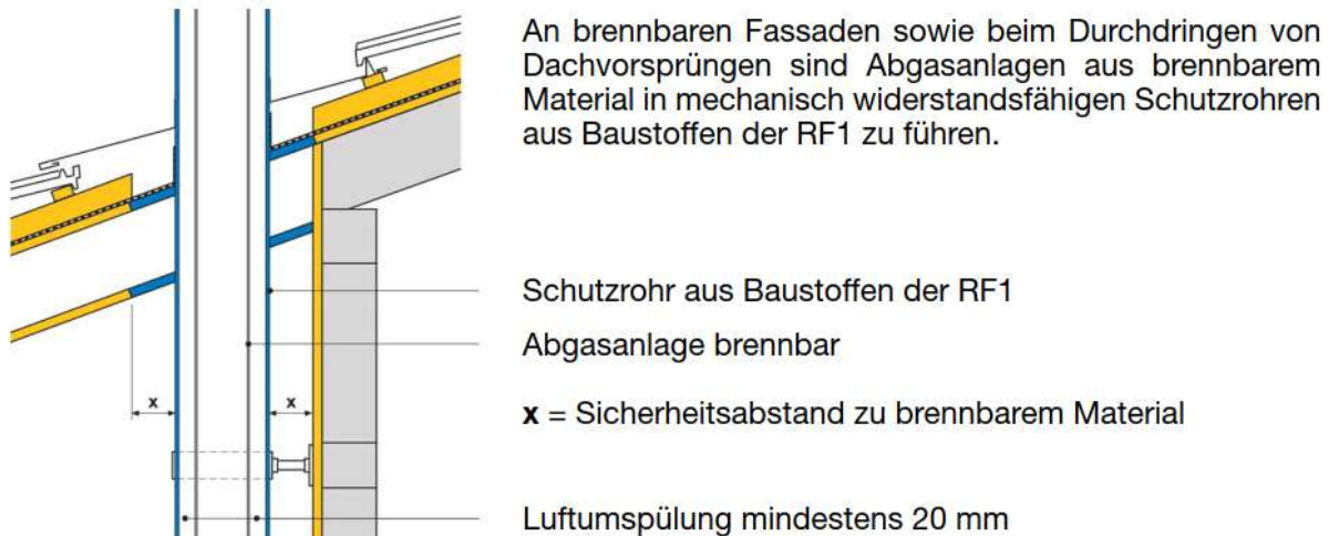
Abb. 81 Führung von Abgasanlagen an Fassaden
