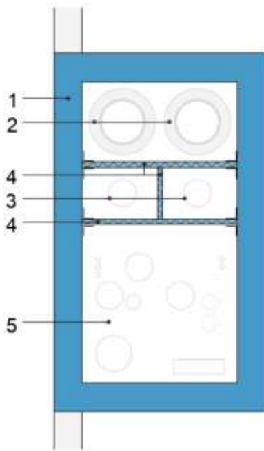
Abb. 31 Vertikale Führung
