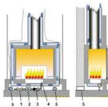
Cheminéeanlage mit LAS und Lüftungsöffnungen
