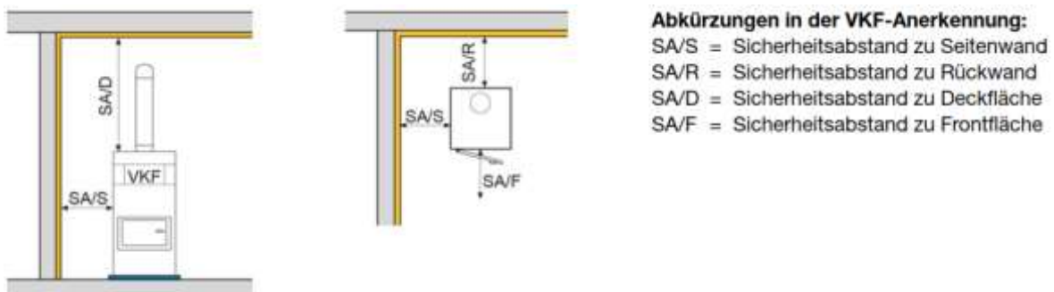
Abb. 35 Sicherheitsabstände
