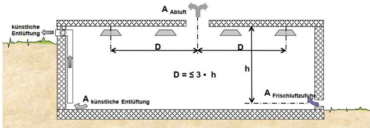
Abb. 87 Abluftöffnung im Dach
