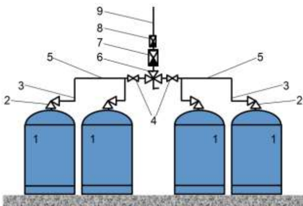
Abb. 21 Mehrflaschenrampe
