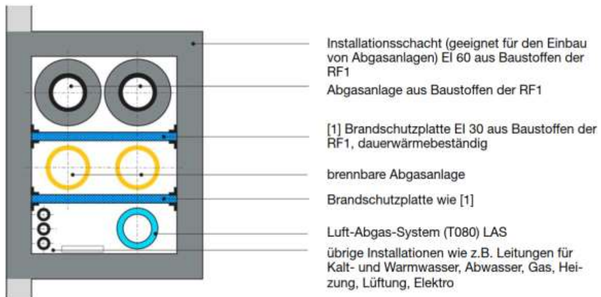
Abb. 80 Führung von Abgasanlagen in Installationsschächten für den Einbau von Abgasanlagen
