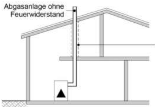
Abb. 77 Beispiel Räume über 2 Geschosse (z.B. Galerie) innerhalb eines Einfamilienhauses oder einer Wohnung
