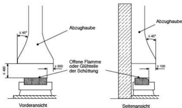
Abb. 85 Massvorgaben zu Abzugshaube an das Gerät angeschlossen und gegen eine nicht brennbare Wand gestellt
