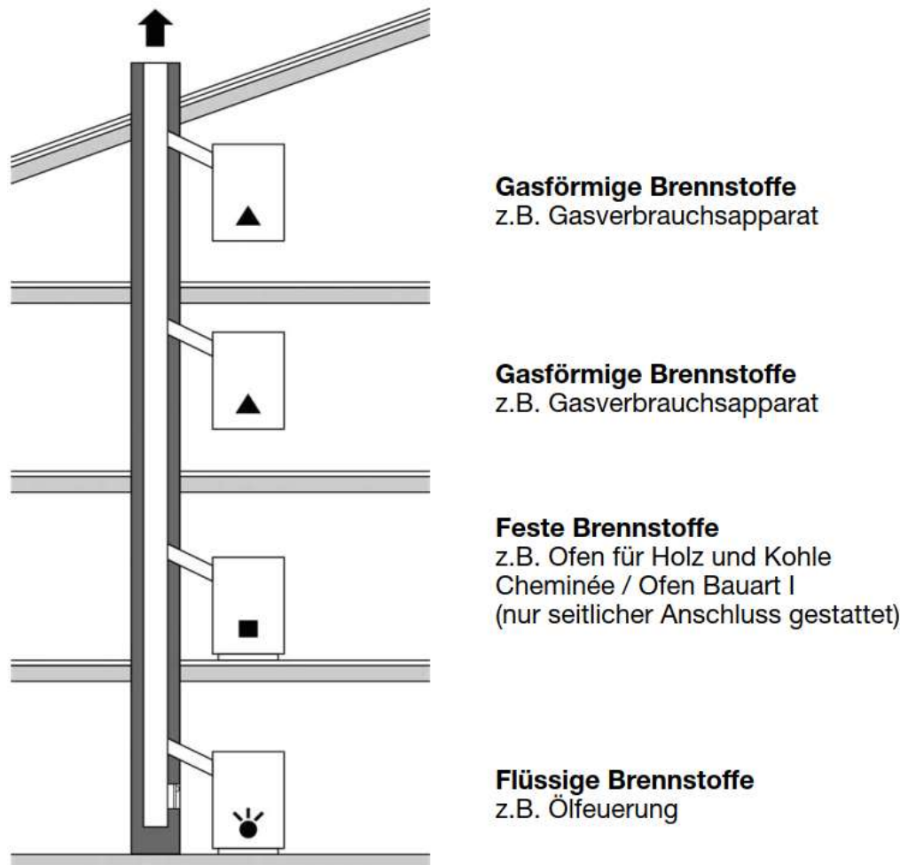
Abb. 61 Mehrfach und/oder gemischte Belegung
