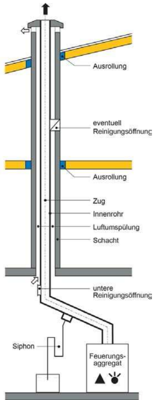
Abb. 58 Abgasanlage im Überdruckbetrieb in Brandschutzelement (Schacht) eingebaut
