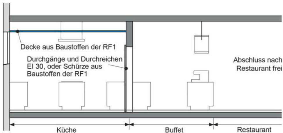
Abb. 46 Küche gegen Buffet abgeschlossen - Buffet ohne Koch- und Grillapparat / Pizzaofen
