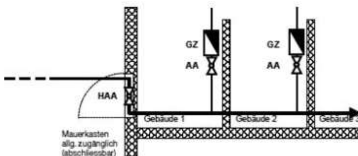
Bezugsquelle: SVGW-Richtlinie G1 für die Erdgasinstallationen in Gebäuden Abb. 27 Absperrarmaturen und Hinweisschilder
