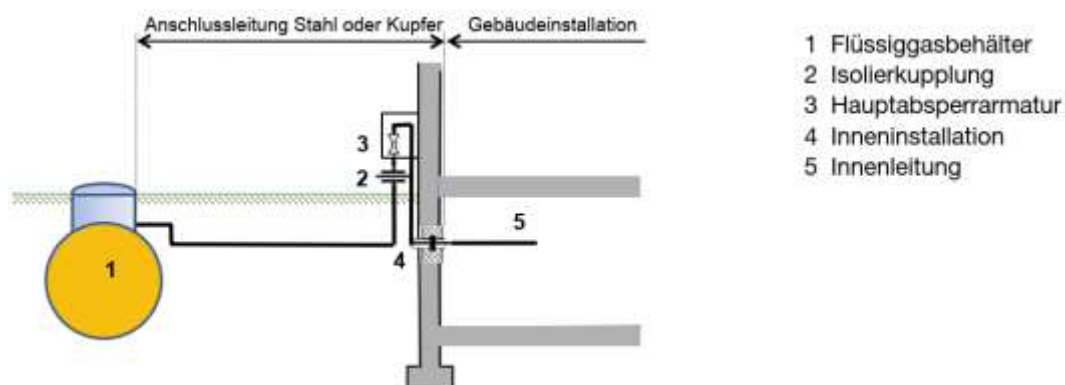
Abb. 24 Anschluss unterflur mit Festpunktsicherung
