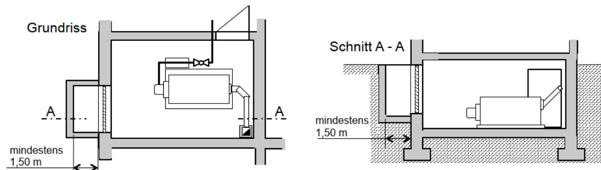
Abb. 43 Druckentlastung
