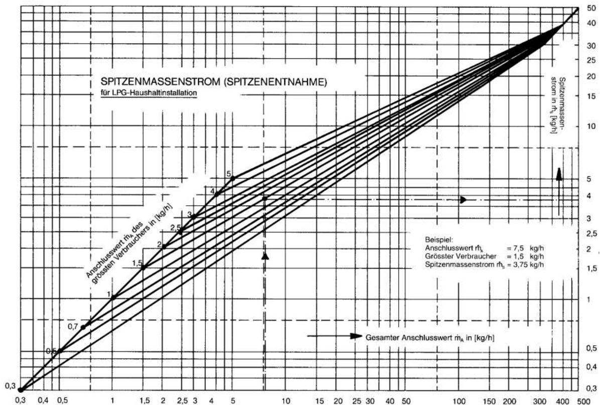
Abb. 34 Diagramm zur Ermittlung des Spitzenmassenstroms (Spitzenentnahme) für Haushaltapparate und Industrielle Kleinverbrauchseinrichtungen
