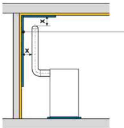
Abb. 74 Beispiel Bekleidung / Brandschutzplatte mit 30 oder 60 Minuten Feuerwiderstand aus Baustoffen der RF1 dauerwärmebeständig = reduzierte Sicherheitsabstände
