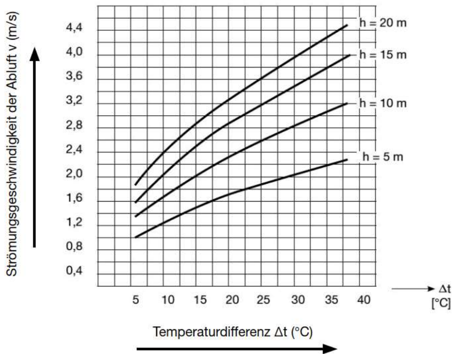
Bezugsquelle: SN EN 13410; gültig für Abluftöffnungen und Abluftleitungen ohne Bögen oder sonstige Hemmnisse Abb. 89 Diagramm Strömungsgeschwindigkeit
