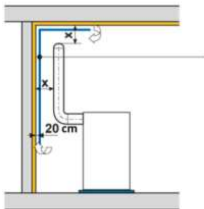
Abb. 73 Beispiel Strahlungsschutz = halbe Sicherheitsabstände
