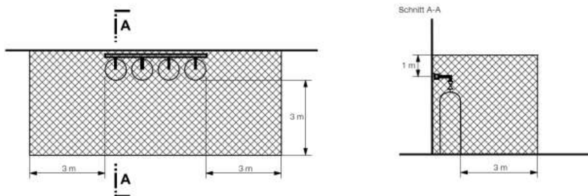
Bezugsquelle Suva-Merkblatt 2153 Abb. 15 Rampe für Transportbehälter
