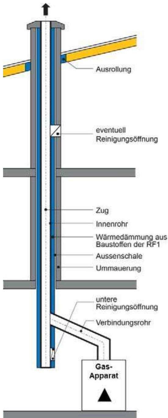
Abb. 57 Abgasanlage im Unterdruckbetrieb in Brandschutzelement (Ummauerung) eingebaut
