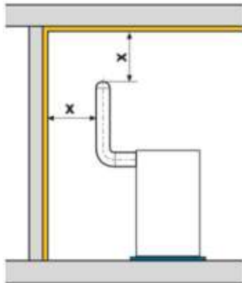
Abb. 72 Beispiel ungeschützt = volle Sicherheitsabstände
