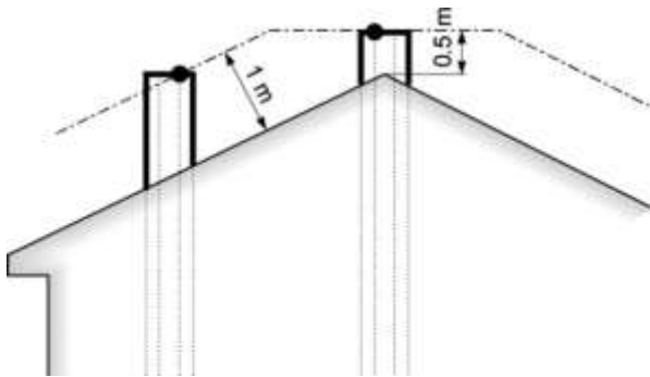
Abb. 64 Beispiel Steildächer
