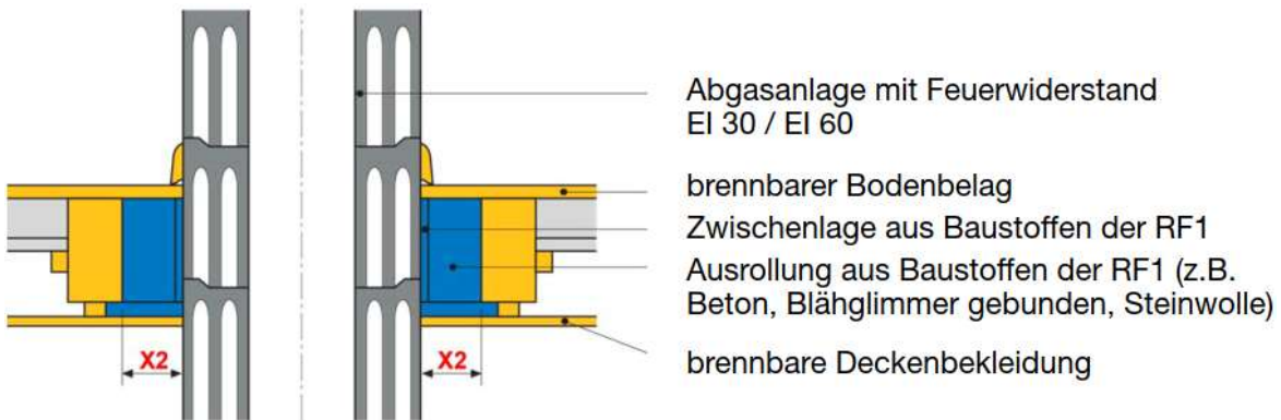
Abb. 71 Durchführung durch Holzdecke - Abgasanlage mit Feuerwiderstand
