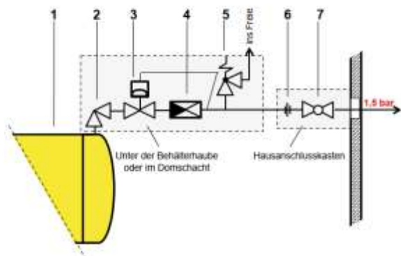
Variante A: Mit SAV und SBV Verteildruck 1,5 bar
