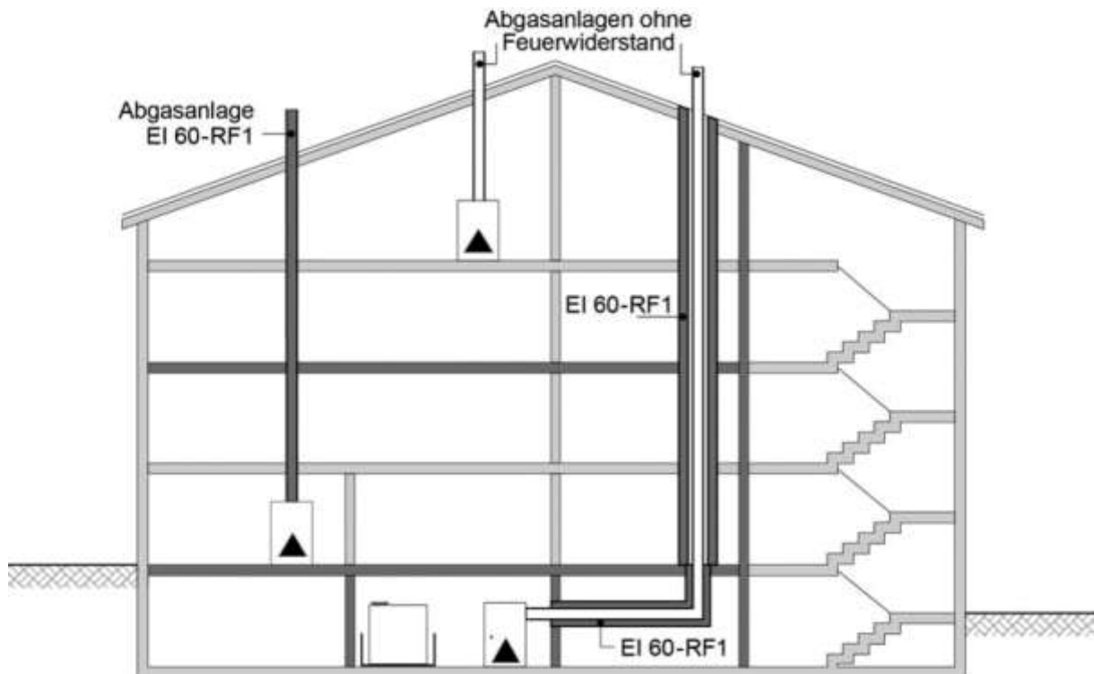
Abb. 79 Beispiel Gebäude mit mehreren Brandabschnitten
