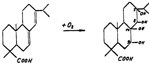
Abbildung 3: Oxidation der Abietinsäure
