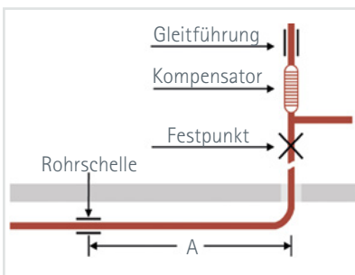
Bild 6.3 Rohrschellenabstand bei Wand- und Deckendurchführungen (4760)
