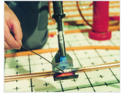
Bild 8.1 Herstellen einer Hartlötverbindung in einer Kupferrohr-Fußbodenheizung (2657)
