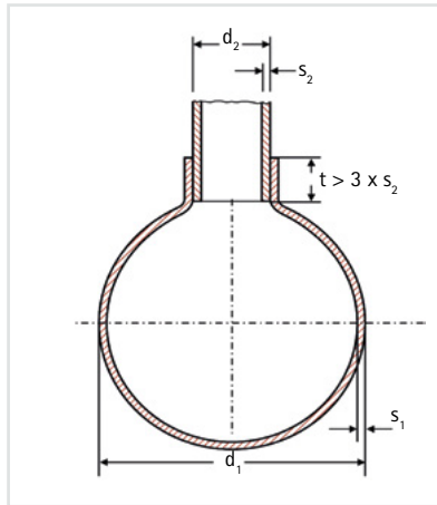
Bild 4.3 Mindesteinstecktiefe bei fittinglos hergestellten T-Abgängen (3569)
