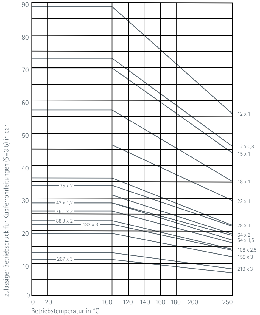
Bild 5.1 Zulässige Betriebsdrücke von Kupferrohrleitungen (Sicherheit S=3,5) in Abhängigkeit von der Betriebstemperatur (3504)
