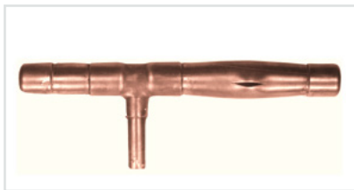
Bild 5.2 Weichgelötete Rohrkombination 22 x 1 mm nach einer Berstdruckprobe von 280 bar (1063)
