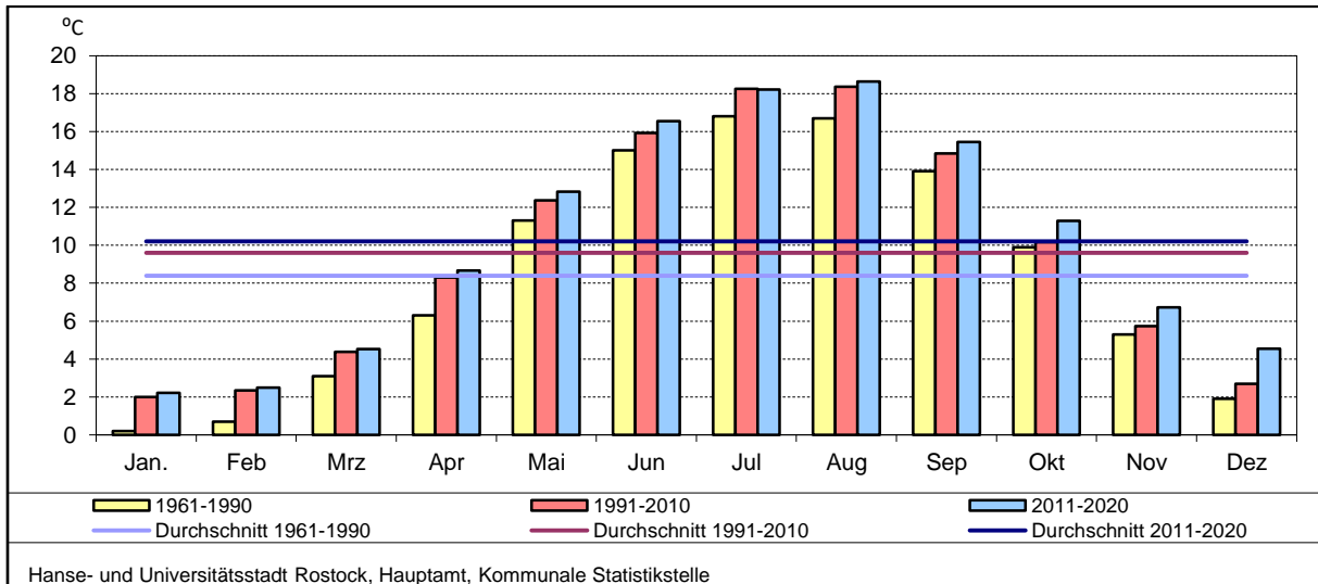
Abb. 1.04 Durchschnittliche Monatssumme der Sonnenscheindauer 1961 bis 2020
