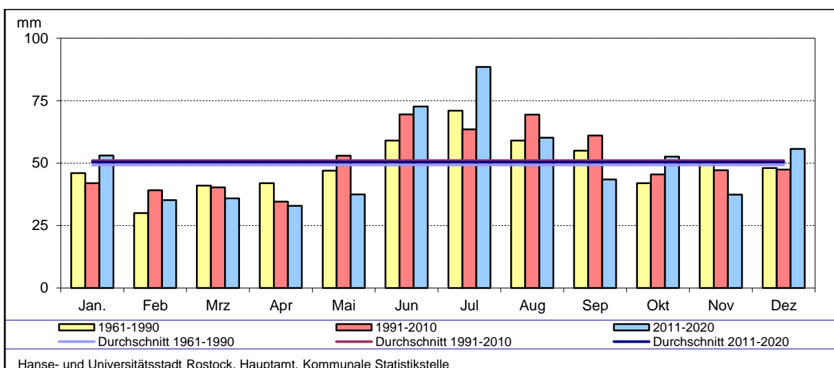
Abb. 1.05 Durchschnittliche Monatssumme der Niederschlagshöhe 1961 bis 2020
