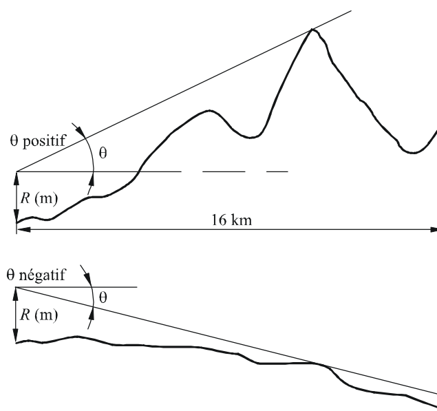
FIGURE A.2.1-3 Angle de dégagement du terrain
