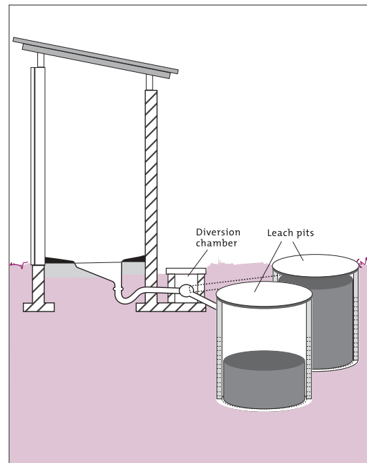
Figure 8.6 Pour-flush latrine
