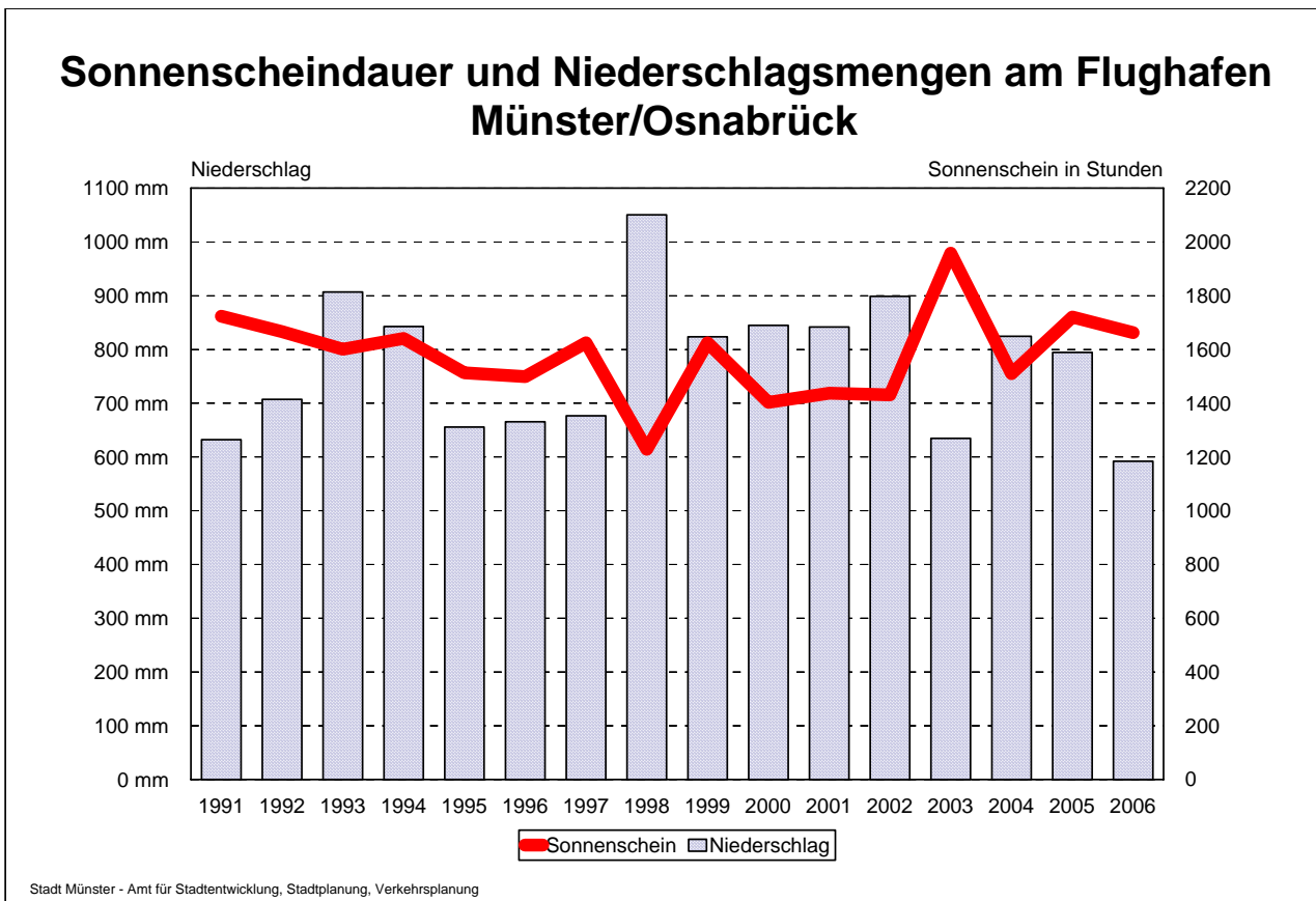
Abbildung 24: Sonnenscheindauer und Niederschlagsmengen am Flughafen Münster/Osnabrück
