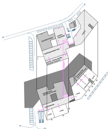
Abb.33 Wettbewerbsergebnis, Sprengzeichnung Brockensammlung, DeZwarteHond
