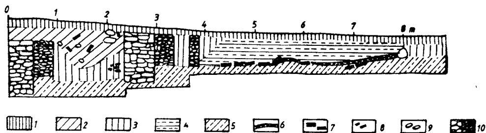
Fig. 7. Tihău. Castrul roman. Clădirea A. Profil parțial din secțiunea II, peretele de sud-vest: 1) sol vegetal; 2) groapă umplută cu moloz și pământ conținând cărămizi și țigle romane fragmentare; 3) pământ de umplutură cu cioburi, bucăți de țigle și cărămizi romane; 4) lentilă de pământ galben cleios, adus și depozitat la fața locului; 5) lut galben neumblat; 6) cocciopesto dislocat din padiment; 7) cărămizi romane; 8) cărbune; 9) pietre de carieră nefasonate; 10) ziduri.
