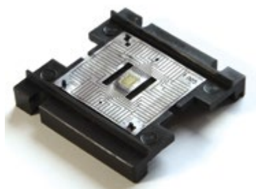
Полиимидный носитель на 48-и выводной рамке
