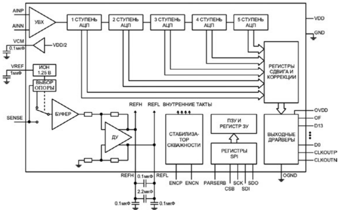
Блок-схема АЦП
