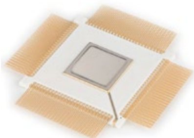
Корпус 4236.208-2
