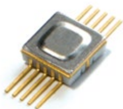
Корпус H02.8-1В
