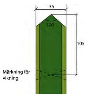
Bild 8.1:2 Vikning av kragsspegel m/58. Måttsättning i mm
