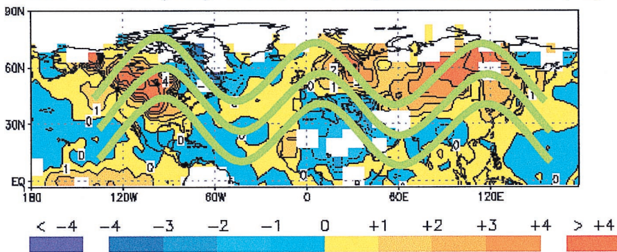
Winter 1991-92 (DJF) Surface Air Temperature Anomalies (°C)
