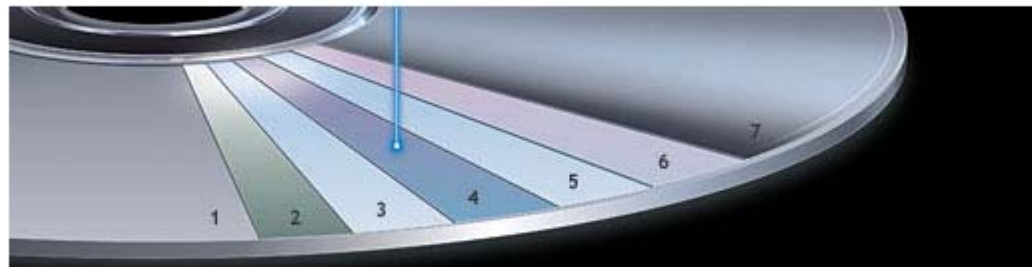
1 Disc substrate 2 Reflective layer 3 Dielectric layer 4 Recording layer 5 Dielectric layer 6 Cover layer 7 DURABIS2 layer
