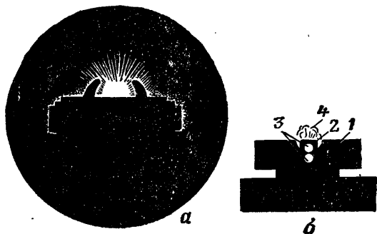
Рис. 86. Прицеливание при стрельбе по цели, обнаруживающей себя вспышками выстрелов: а — с помощью предохранителя мушки и прицельной планки; б — с помощью приспособления для стрельбы ночью; 1 — целик; 2 — мушка; 3 — светящиеся точки; 4 — вспышки выстрелов
