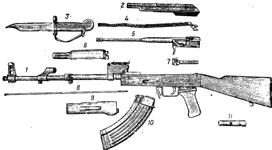
Рис. 2. Основные части и механизмы автомата:
