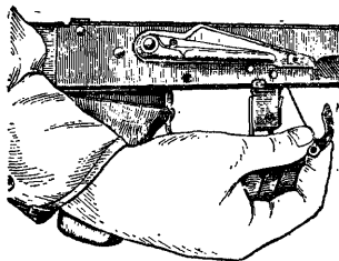
Рис. 18. Извлечение авто-спуска с пружиной из ствольной коробки
