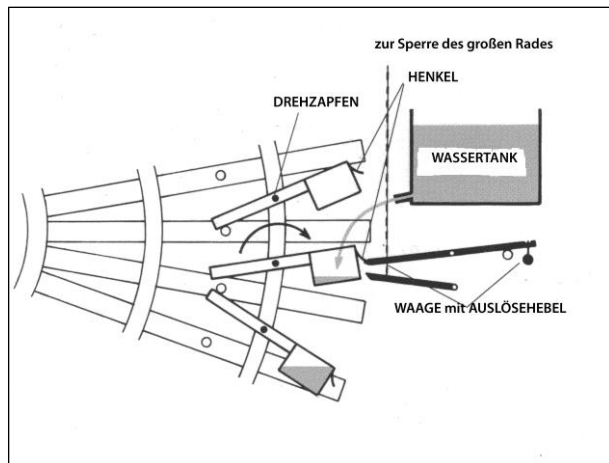
Stop-and-Go-Hemmungsmechanismus der großen, von einer Wasseruhr getriebenen astronomischen Simulation des Sü Song, China, 11. Jahrhundert
