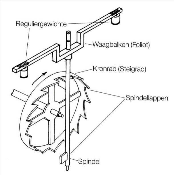
Mechanische Uhrwerkhemmung, sog Waagbalckenhemmung, entwickelt in Europa Ende des 13. Jahrhunderts
