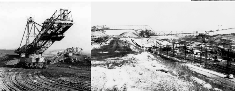
Geräteverbund mit Schaufelradbagger im Tagebau Profen, 1973 Abraumförderbrückenverband, bestehend aus den AFB F32-16 und F34-26 im Tagebau Profen-Nord, um 1980
