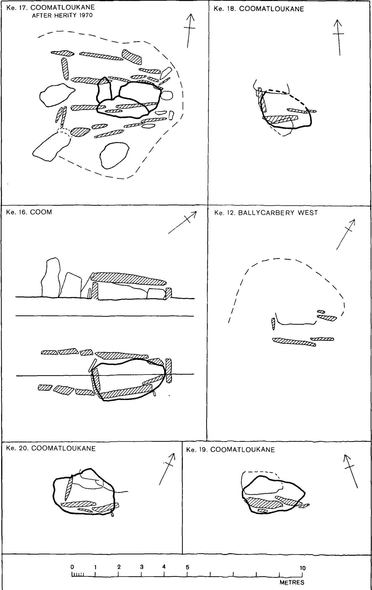
Fig. 25 Wedge Tombs Co. Kerry
