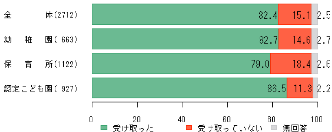
図 18 通知の受取
