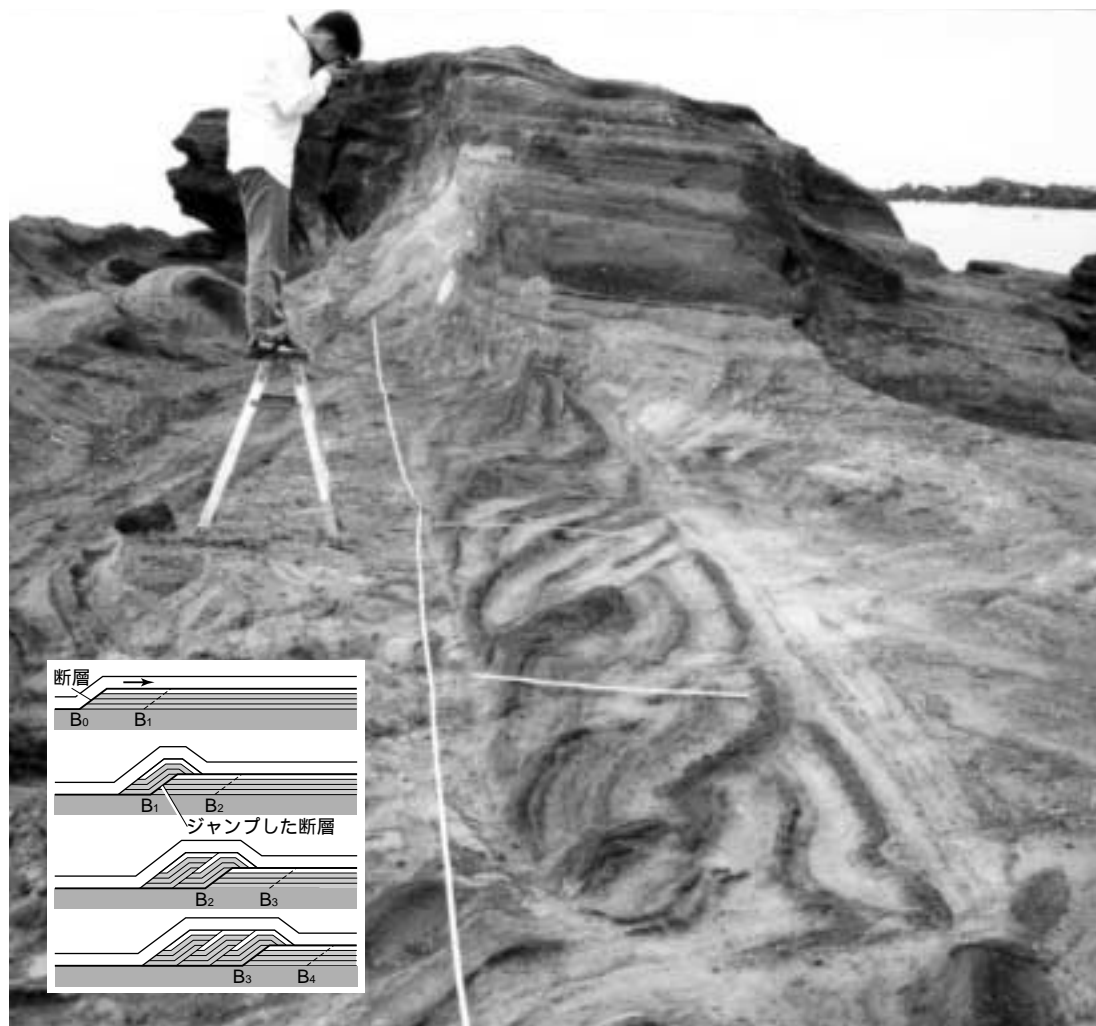
三浦層群三崎層( 新生代第三紀中新世後期～鮮新世前期 )に見られるデュプレックス構造( 神奈川県三浦市黒鯛込 )
