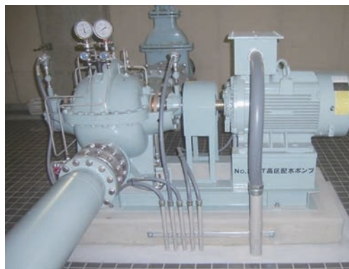
インバータ制御方式のポンプ インバータ制御によりポンプの流量を調整することで、効率の良い運転を行うことができます。
