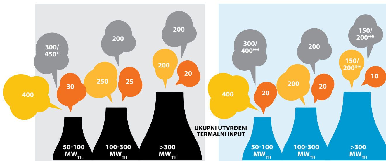
Slika 2. Granične vrednosti emisije za postojeća i nova postrojenja u kojima se lože ugalj, lignit i druga čvrsta goriva prema IED. Blokovi u svim slučajevima: mg/Nm 3 . SO 2 NO x PRAŠINA
