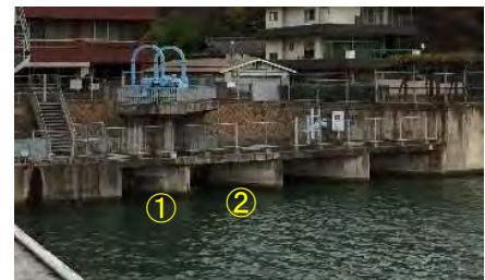
左岸下流側 ①魚道ゲート、②ロック式魚道
