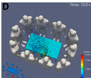
SIMULAÇÃO DE TOSSE EM LOCAL ABERTO COM BRISA. SEM DISTANCIAMENTO E SEM MÁSCARA.
