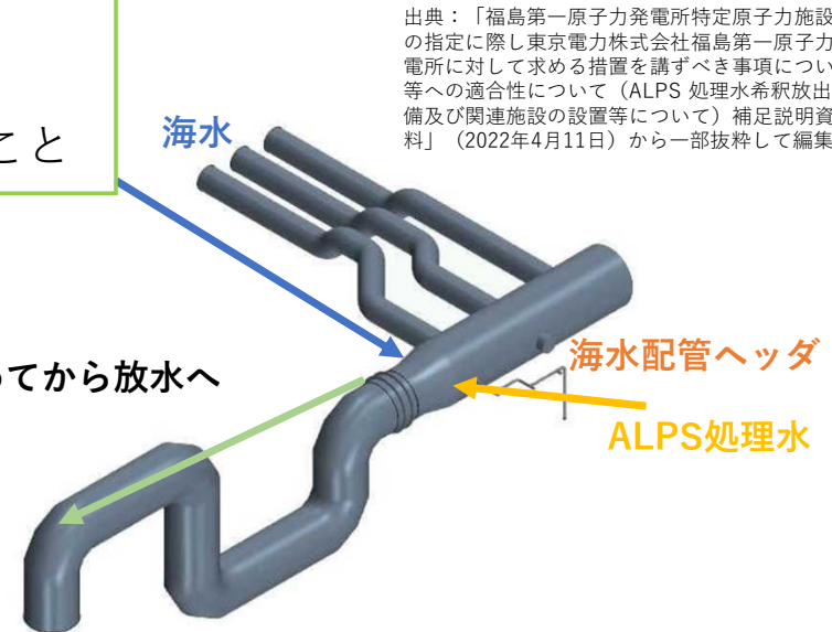
図：海水配管ヘッダ等の解析モデル
