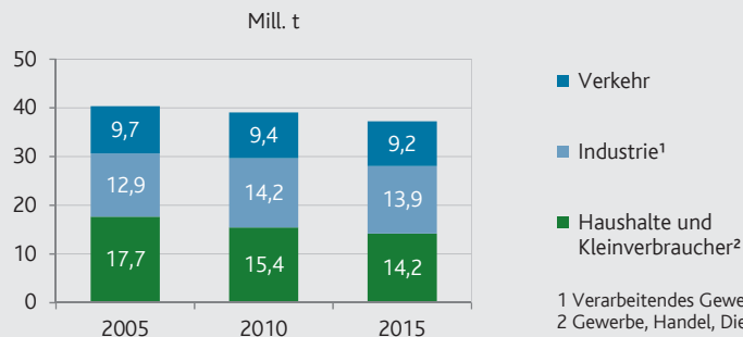
G 10 CO 2 -Emissionen aus dem Endenergieverbrauch (Verursacherbilanz) 2005–2015 nach Emittentensektoren
