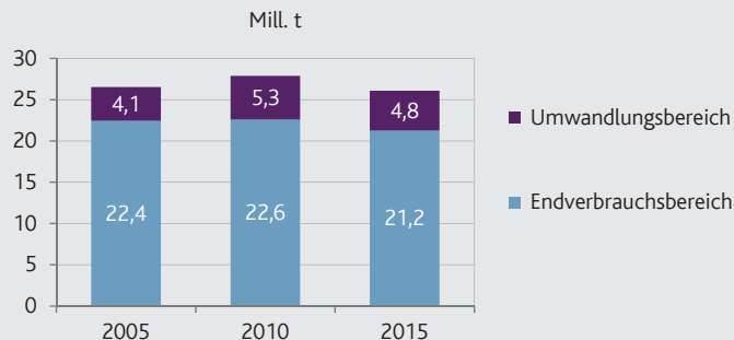
G 8 CO 2 -Emissionen aus dem Primärenergieverbrauch (Quellenbilanz) 2005–2015 nach Emittentensektoren
