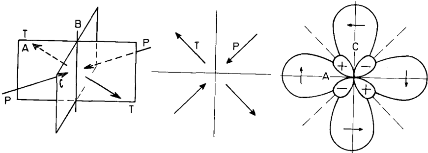
Abb. 3: Links: Hauptspannungsachsen (max. Druckspannung P, max. Zugspannung T und intermediäre Achse B) und Herdflächen (Bruchfläche A, Hilfsfläche C); mitte: im Grundriß; rechts: Polardiagramm der Amplituden der P-Wellen (innen) und der S-Wellen (außen); die Knotenlinien A und C trennen die Quadranten mit Kompressions (+) und Dilatationseinsätzen (-).
